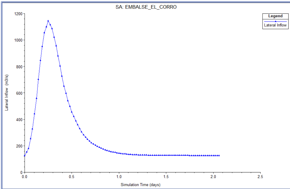
Figura N° 28. Hidrograma para la Apertura Súbita de Compuertas con periodo de retorno 1 en 50 años.
