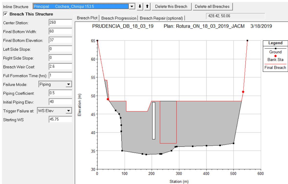
Figura N° 23 Esquema de Rompimiento de Presa El Corro
