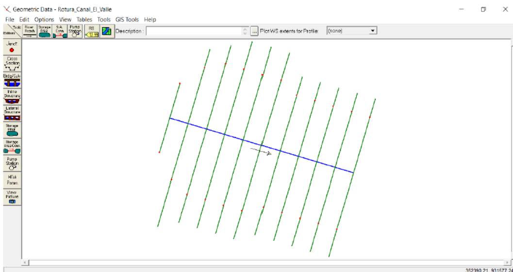
Figura N° 27 Esquema del Modelo HEC-Ras aguas debajo del rompimiento del Canal
