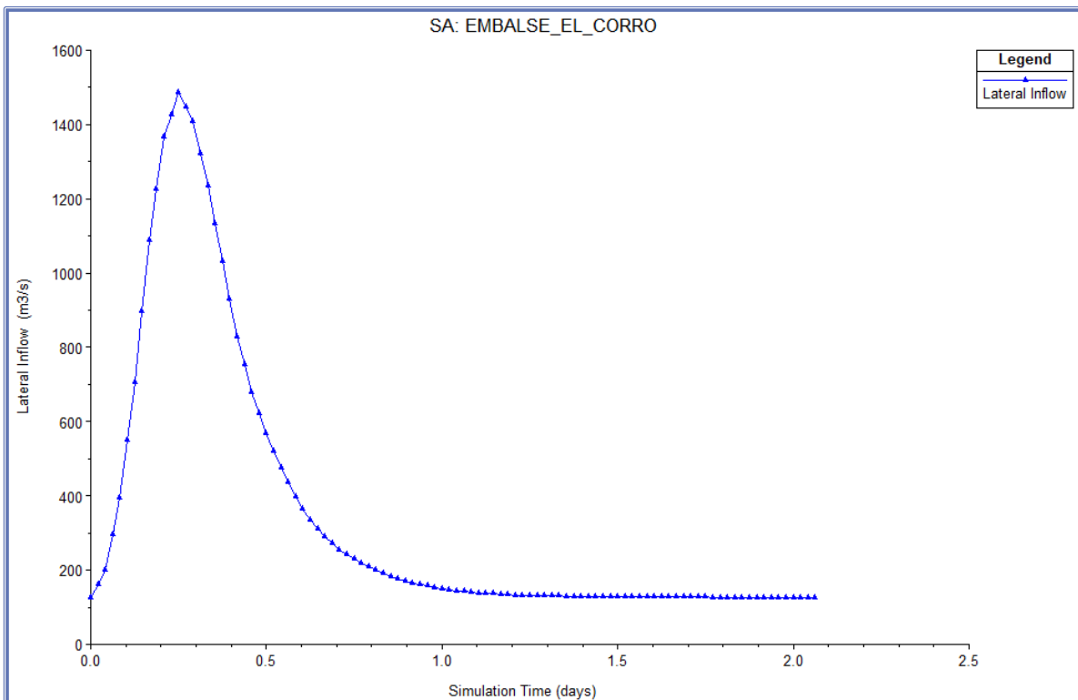
Figura N° 22. Hidrograma de Crecida Extraordinaria para un periodo de retorno 1 en 1000 años
