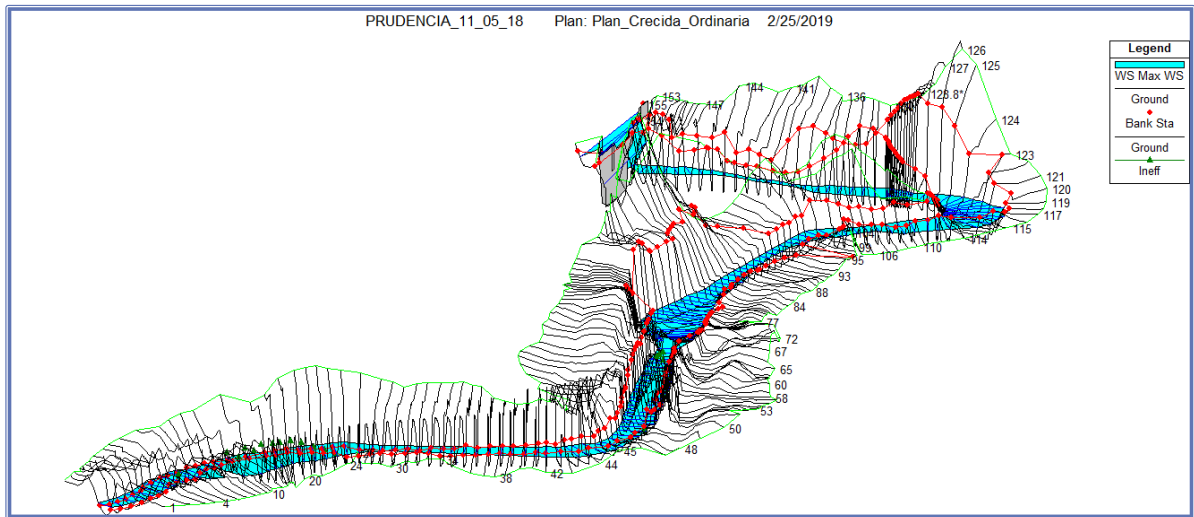
Figura N° 20. Vista en tres dimensiones del modelo de la Presa El Corro, con las secciones transversales del Canal de Aducción.
