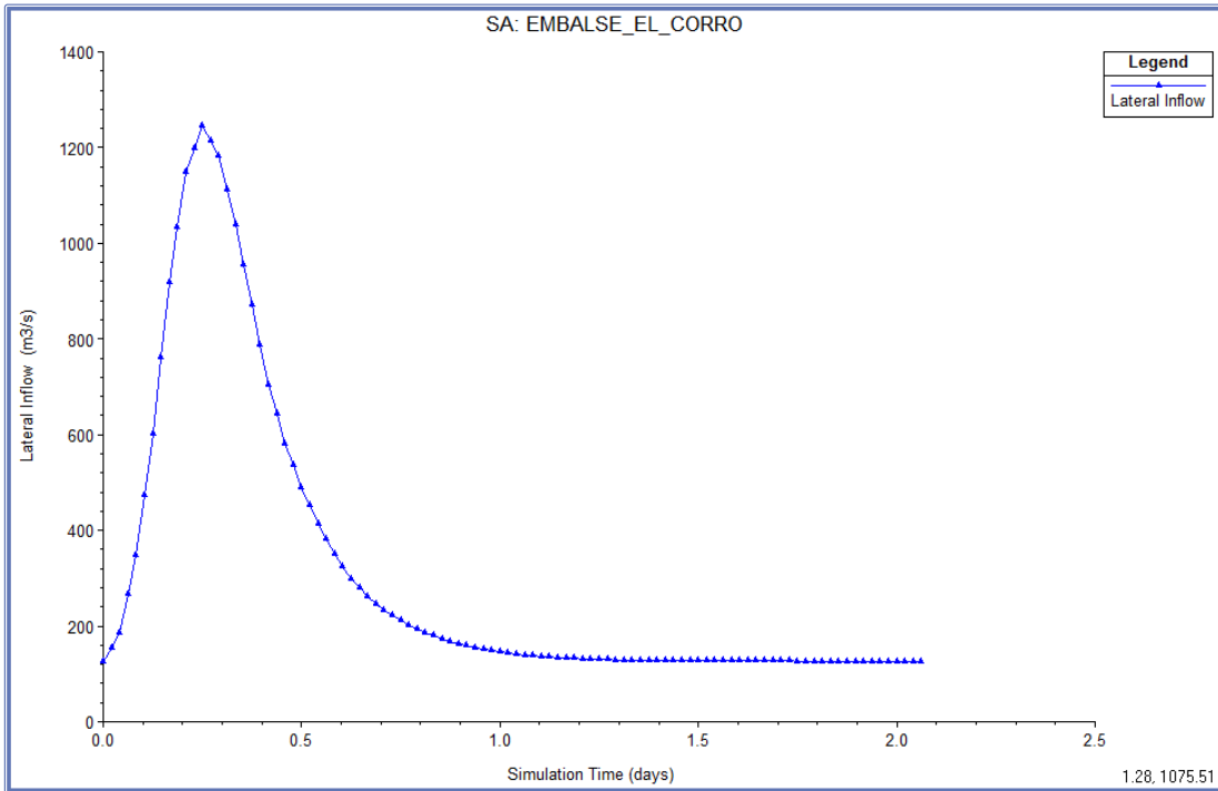
Figura N° 21. Hidrograma de Crecida Ordinaria para un periodo de retorno 1 en 100 años Los resultados de la modelación para la crecida ordinaria se presentan en la Tabla N° 11.
