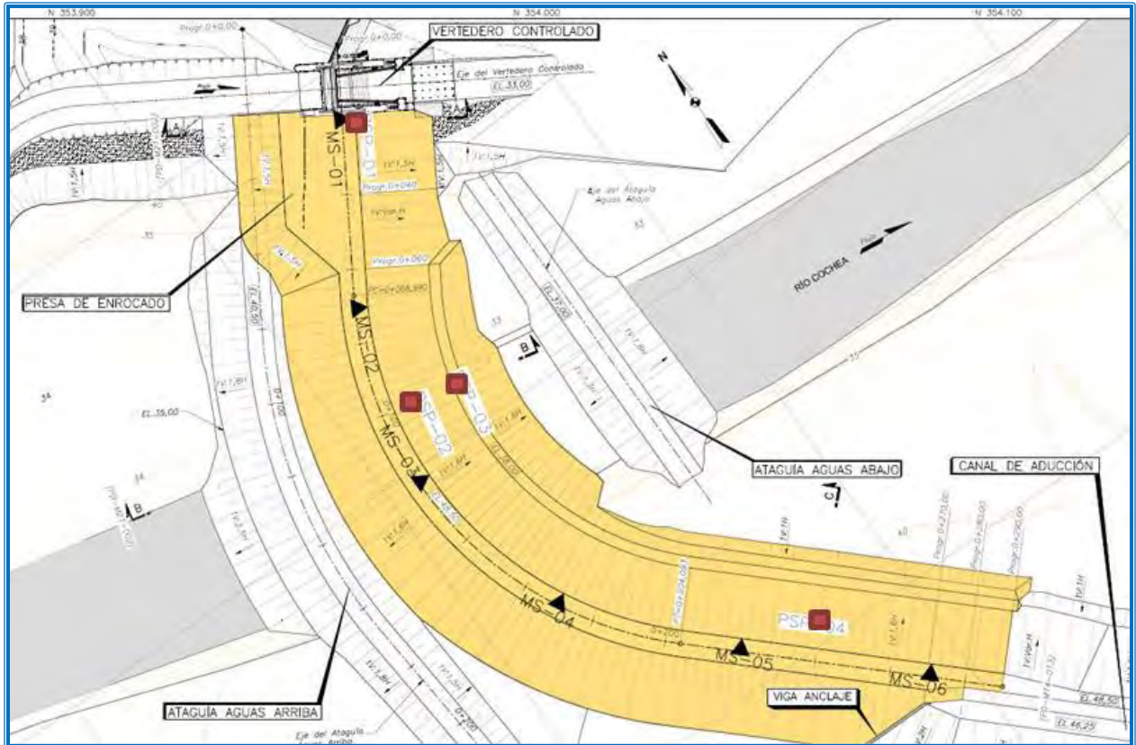
Figura N° 14: Ubicación de los marcos superficiales y piezómetros en la presa El Corro – sección A-A.
