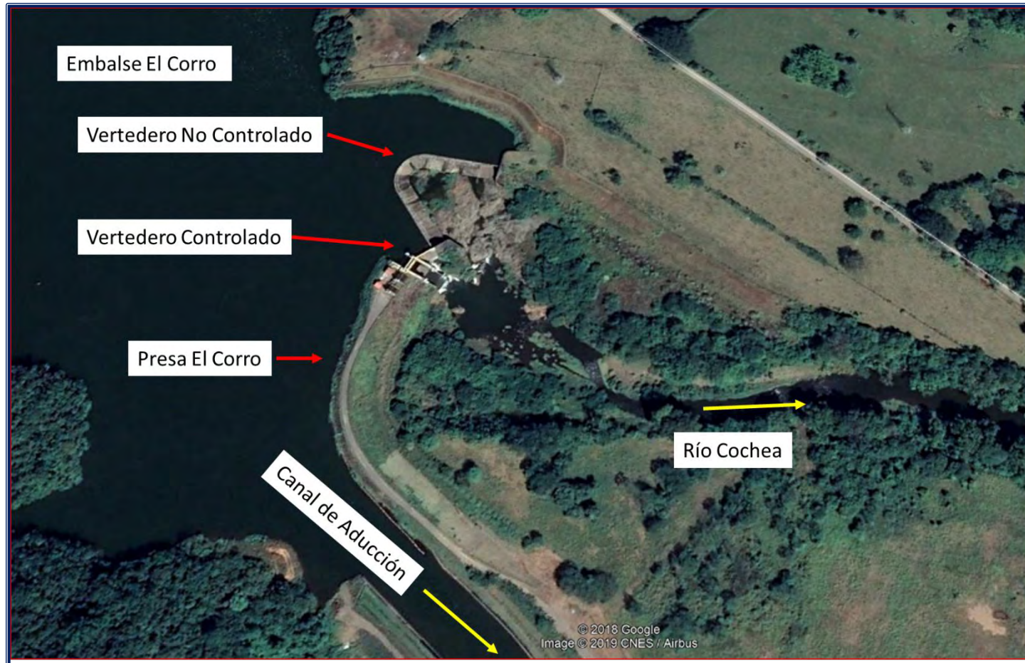
Figura N° 6: Vista de planta de la Presa El Corro y sus componentes principales. Fuente Google Earth.
