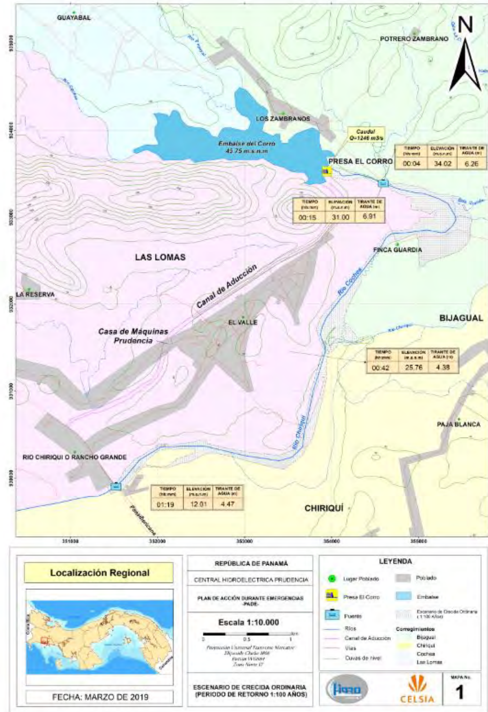
ESCENARIO DE CRECIDA ORDINARIA (PERIODO DE RETORNO 1:100 AÑOS)
