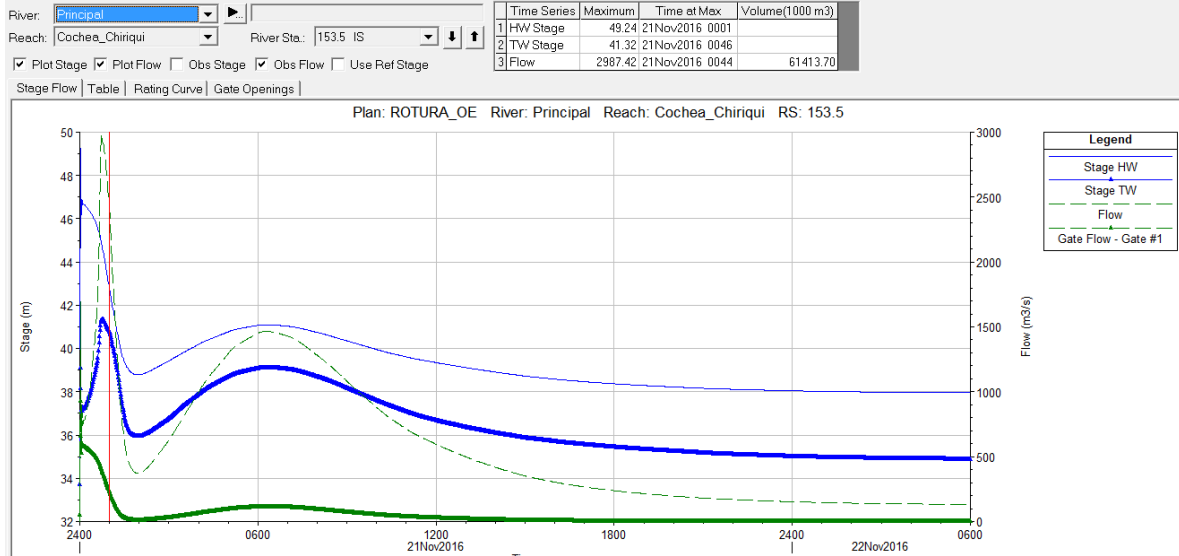
Figura N° 25. Hidrograma de Salida de la Rotura de Presa El Corro en Condición de Operación Extraordinaria
