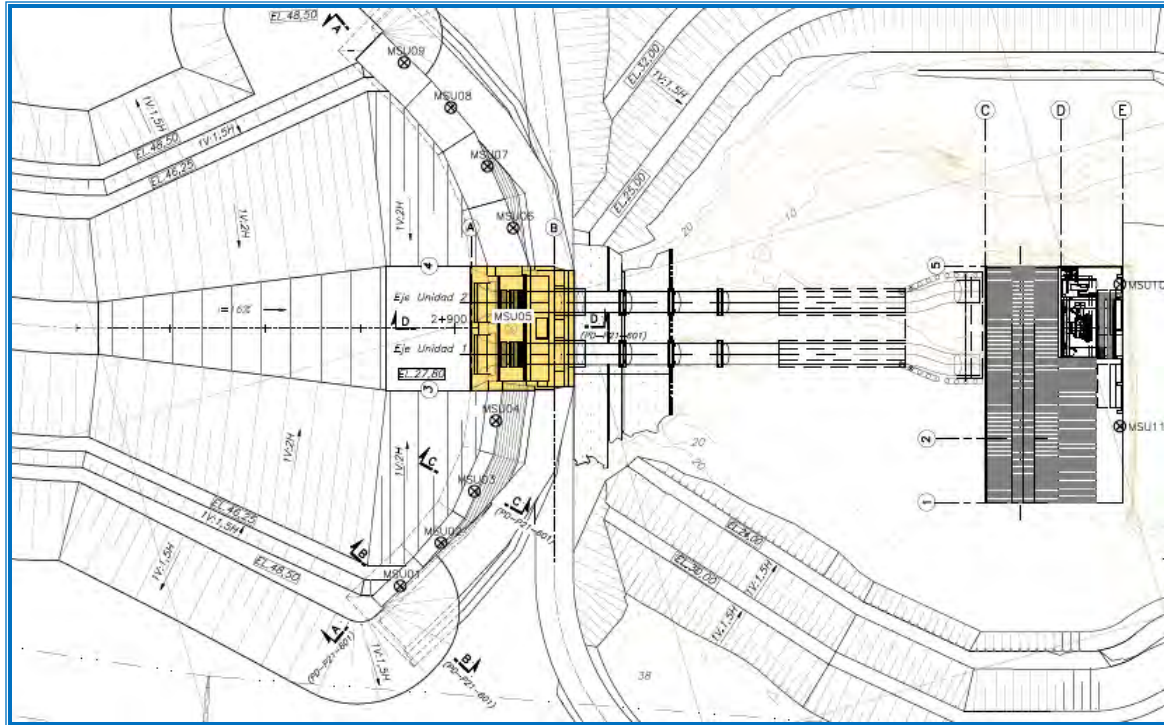
Figura N° 15: Ubicación de los marcos superficiales y piezómetros en la presa El Corro- Sección B-B.
