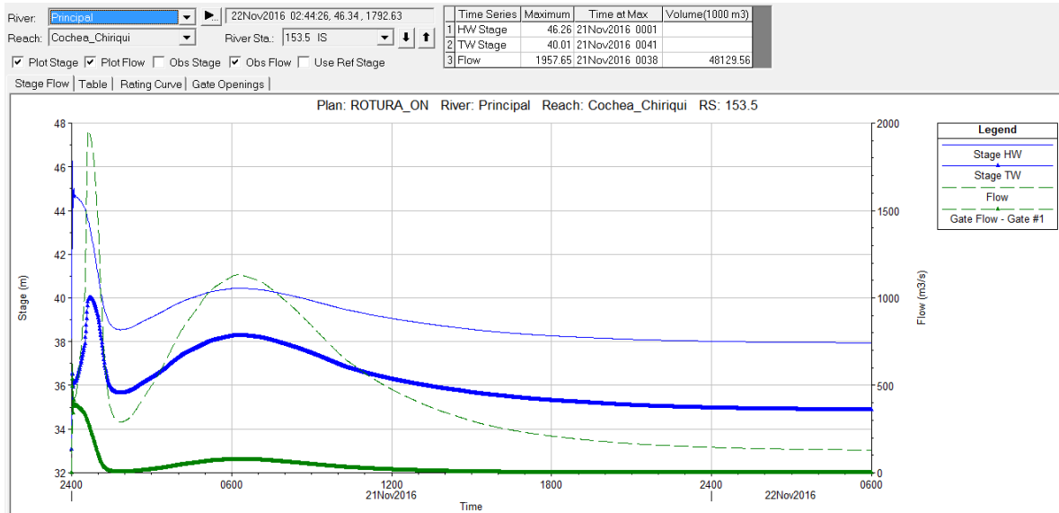
Figura N° 24. Hidrograma de Salida de la Rotura de Presa El Corro en Condición de Operación Normal
