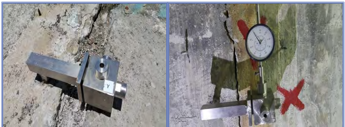
Figura N° 11: Medidores tri-ortogonales de junta de galerías y cresta de Boca de Toma de Prudencia. Fuente: Alternegy, S.A.
