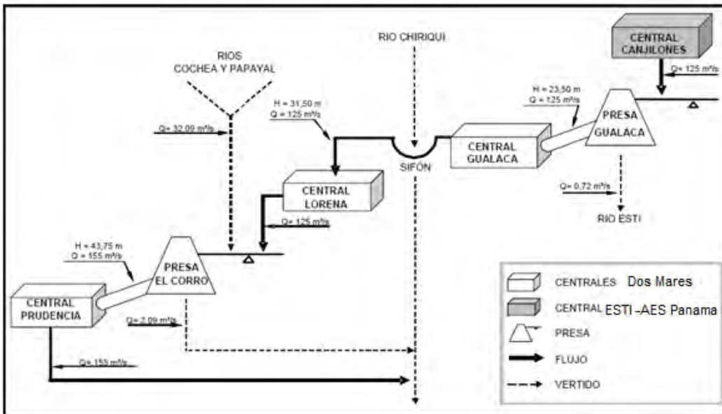
Figura N° 4 Esquema Hidráulico del Complejo Hidroeléctrico Dos Mares. Fuente Consultor
