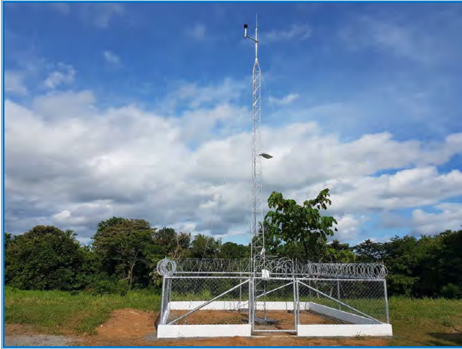
Figura N°17. Estación Meteorológica de la CH Prudencia. Fuente. Alternegy.
