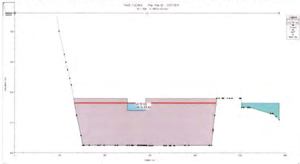
Figura N° D10 - Escenario 0: Secciones transversales de la presa Cochea
