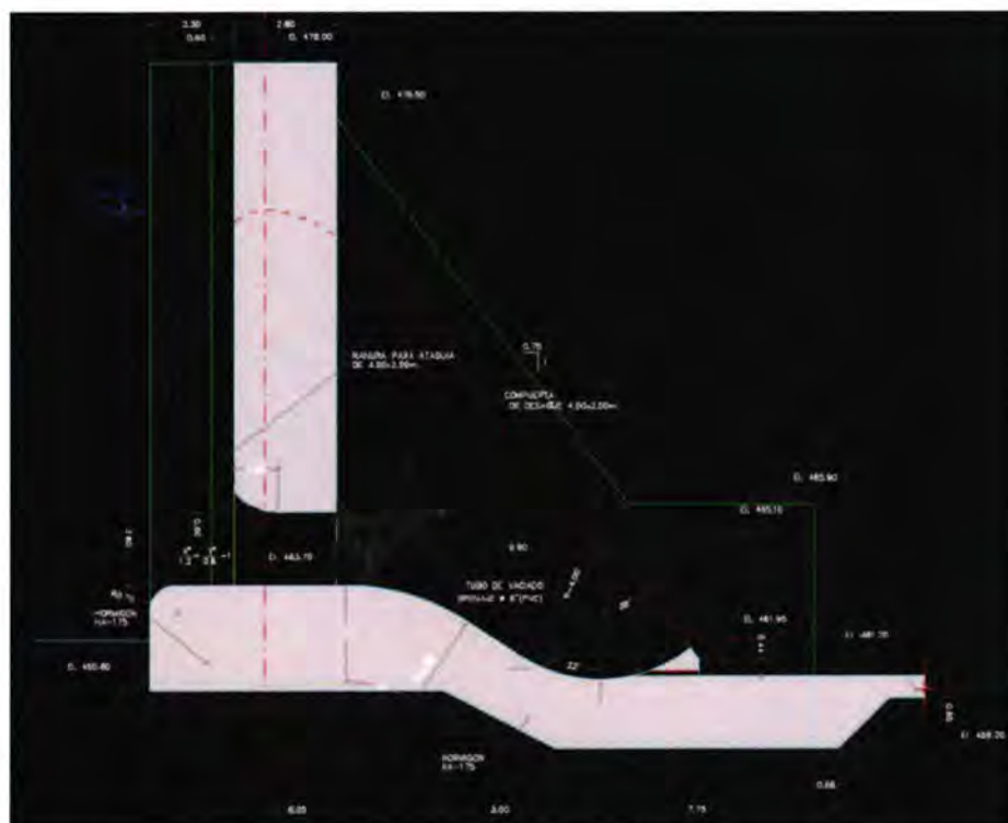
Figura N°5 –Perfil de la descarga de fondo de la presa Cochea
