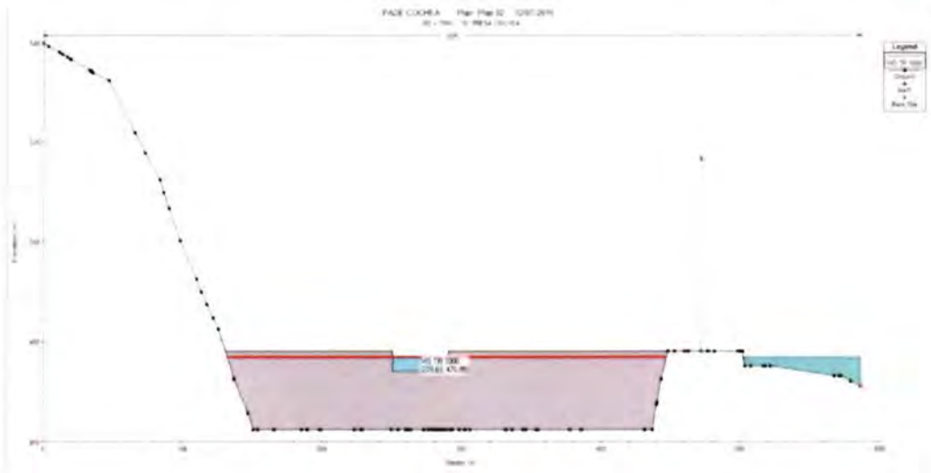
Figura N° D14 - Crecida en el sitio de presa Cochea
