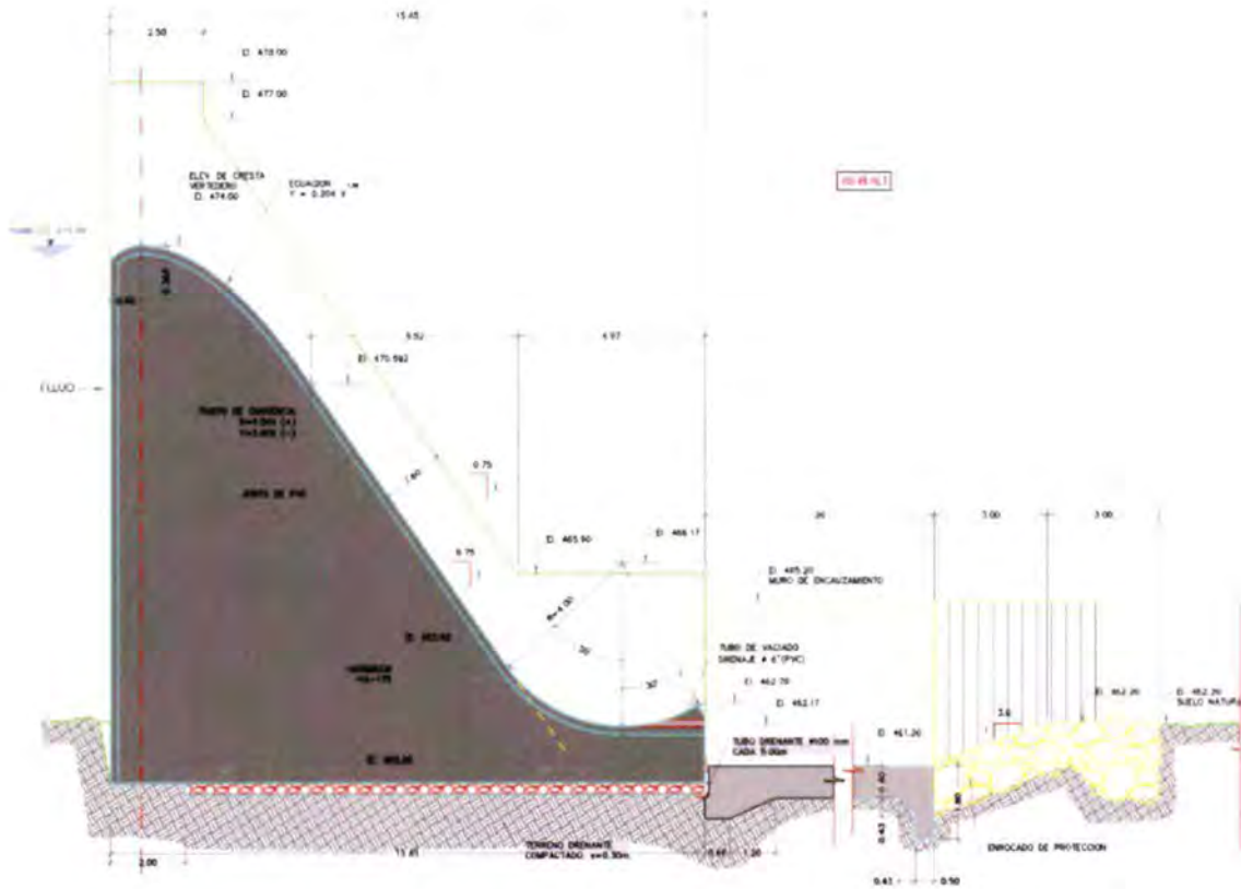
Figura N°6 –Perfil de la presa Cochea por el vertedero
