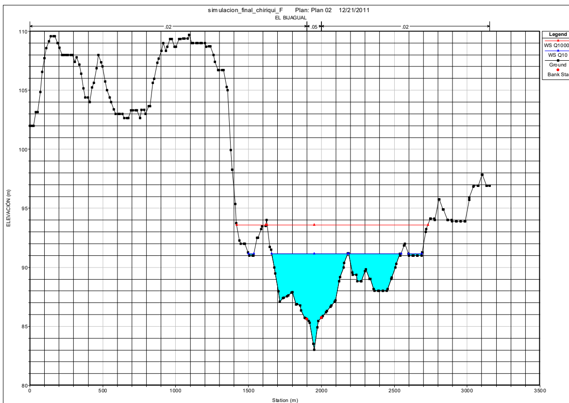
Figura 11: Sección transversal 13 K + 600, vista transversal de la comunidad El Bijagual 30
