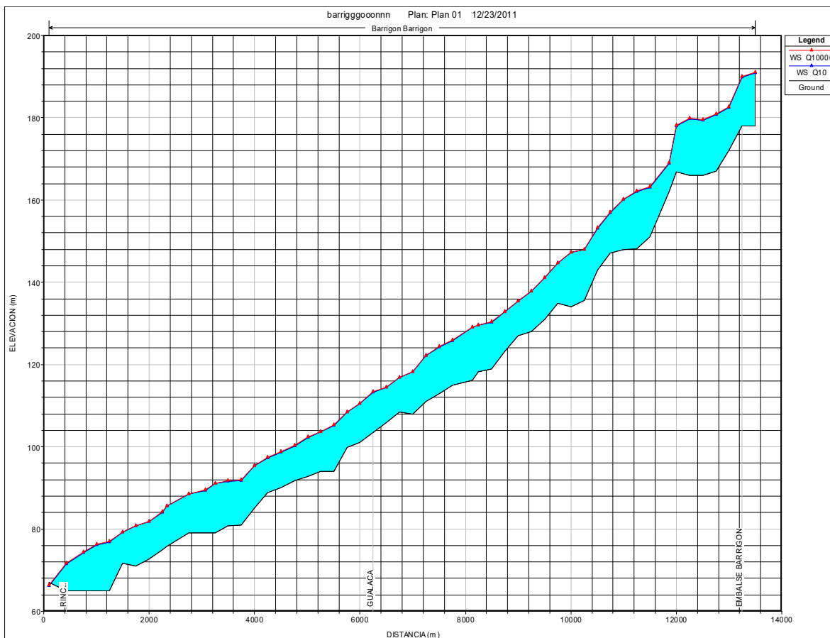
Figura 13: Perfil longitudinal Río Chiriquí desde La Presa Barrigón 32
