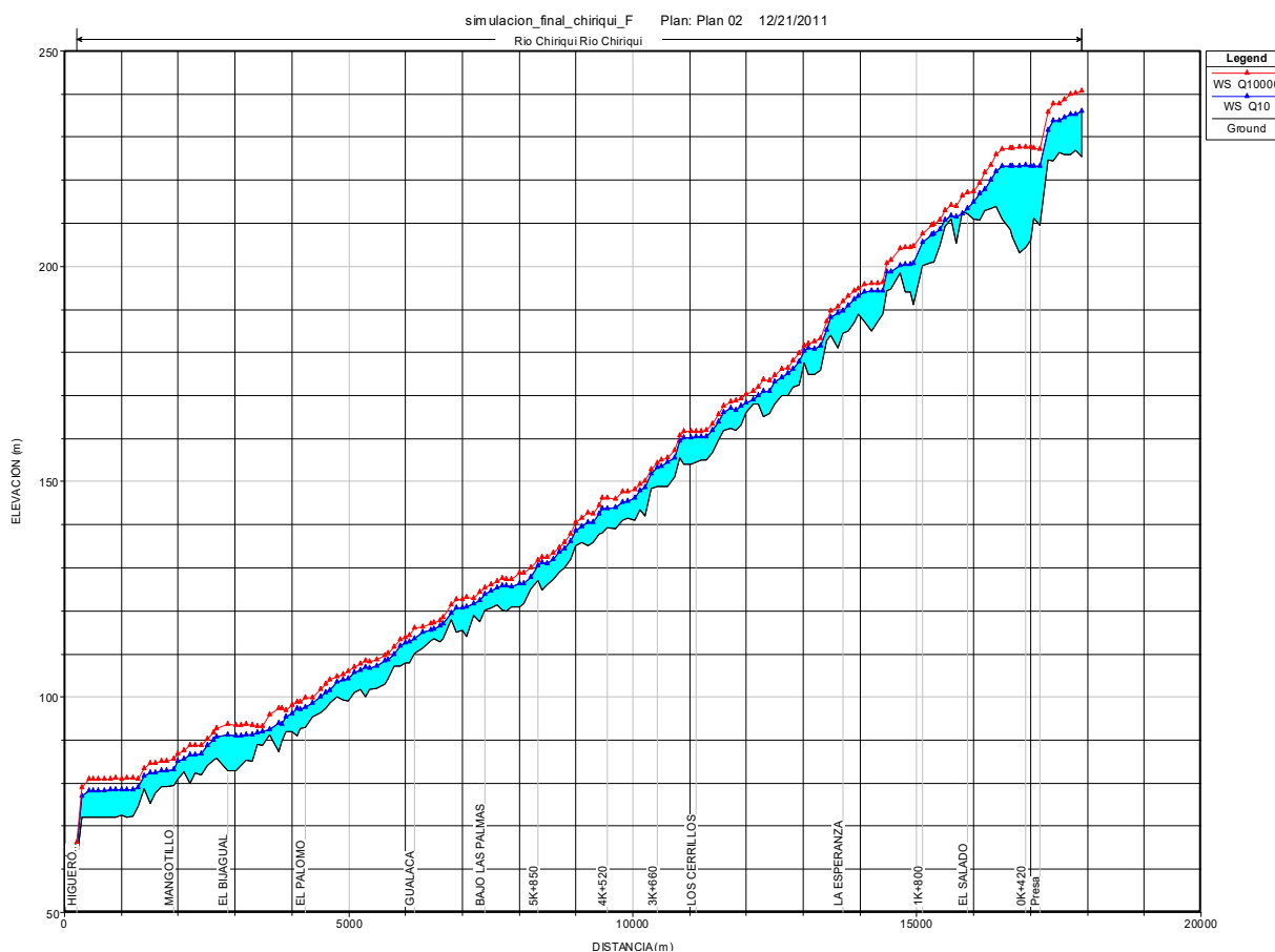
Figura 5 Perfil longitudinal Río Chiriquí desde La Pesa Chiriquí 24
