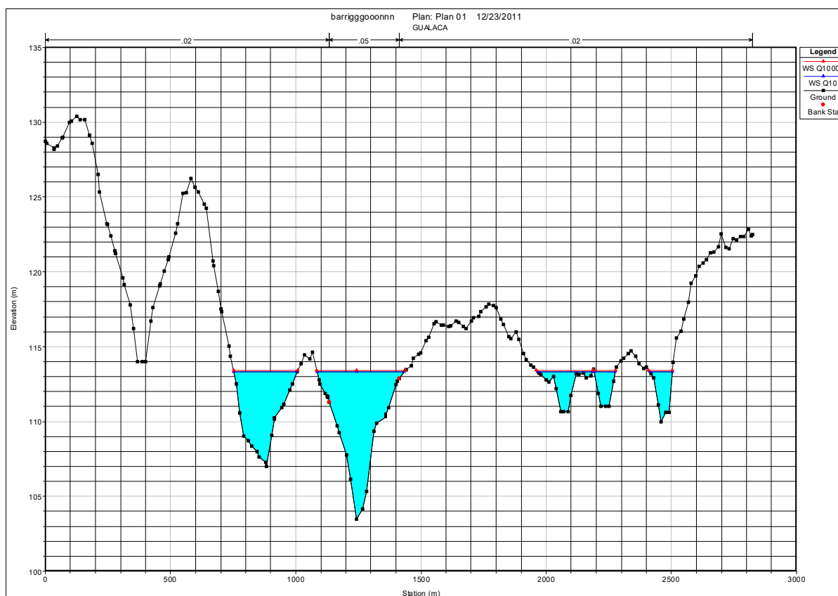
Figura 14: Sección transversal de la comunidad de Gualaca para la simulación desde la presa Barrigón 33
