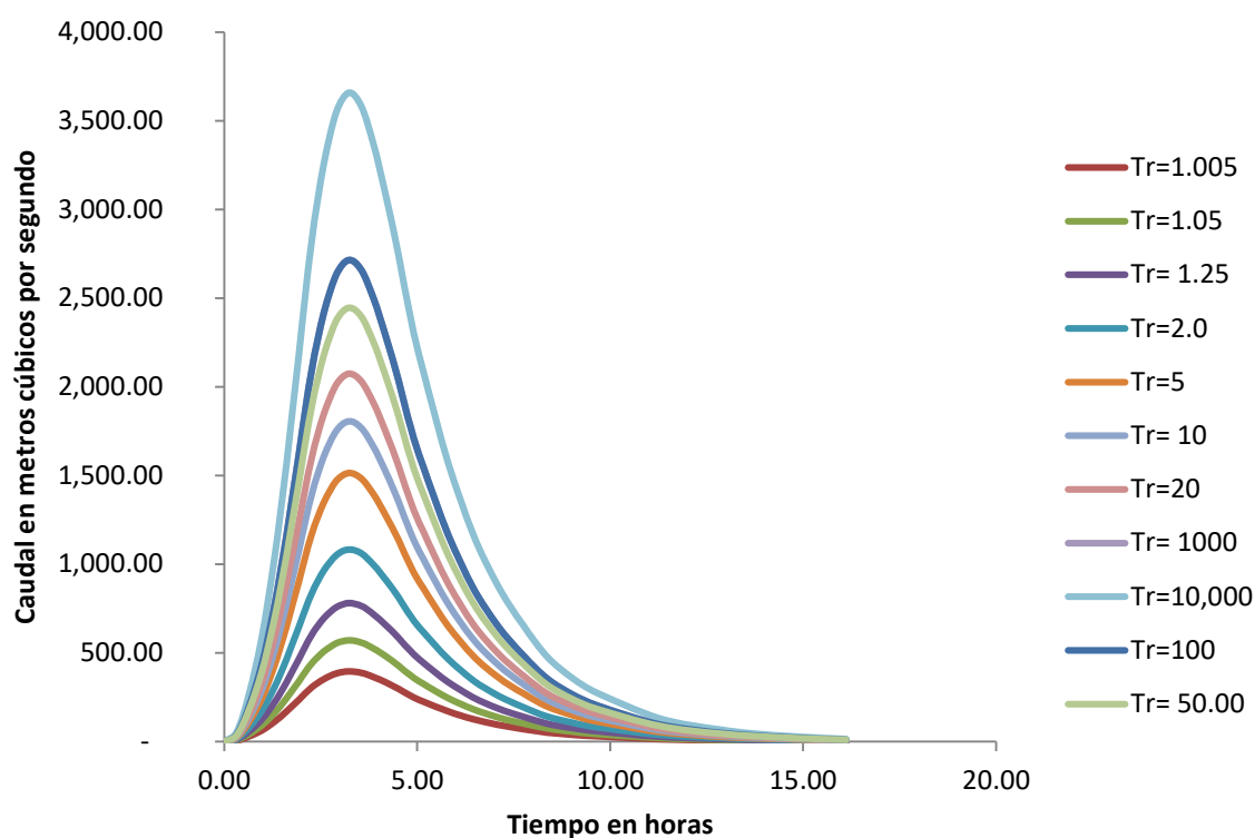
Figura 3. Curvas de caudales con diferentes periodos de retorno presa sobre el río Chiriquí 15
