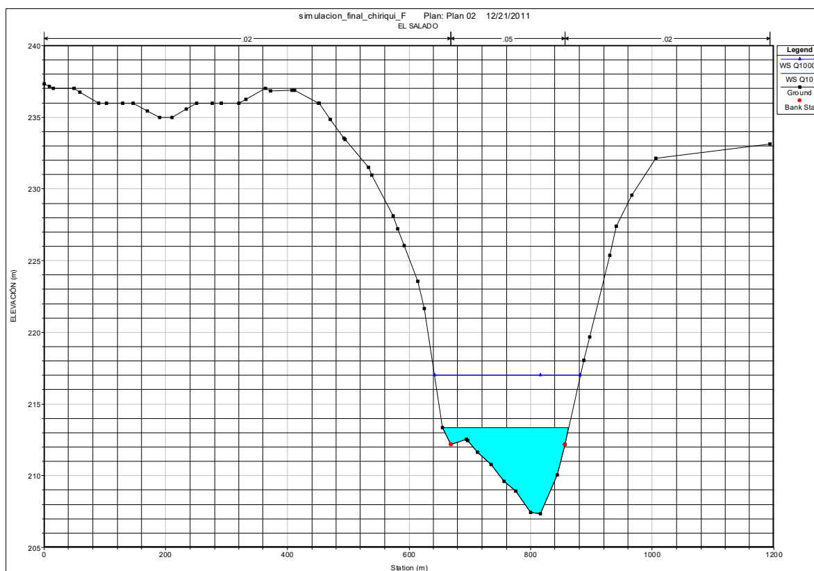
Figura 6: Sección transversal 1K+ 060, vista transversal de la comunidad El Salado 25
