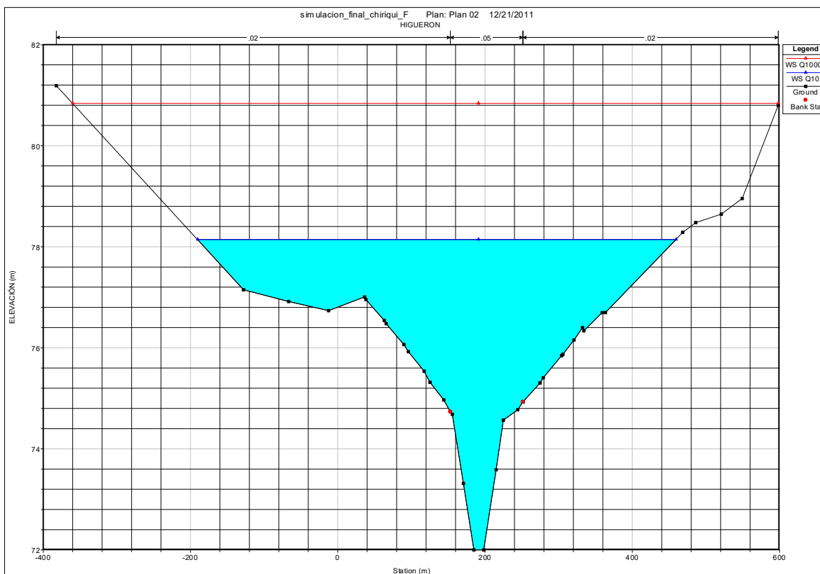
Figura 12: Sección transversal 16 K + 030, vista transversal de la comunidad El Higuérón 31
