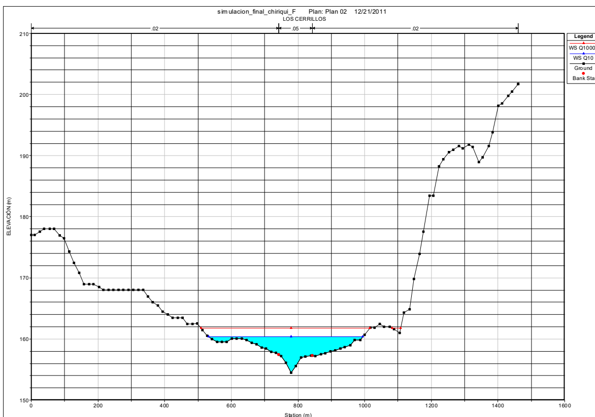
Figura 8: Sección transversal 2 K + 860, vista transversal de la comunidad Los Cerrillos 27
