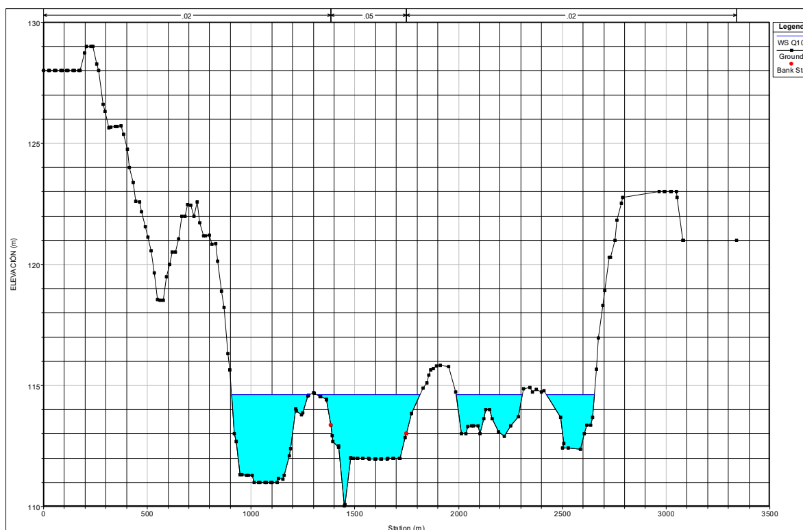
Figura 9: Sección transversal 10 K + 700, vista transversal de la comunidad Gualaca 28
