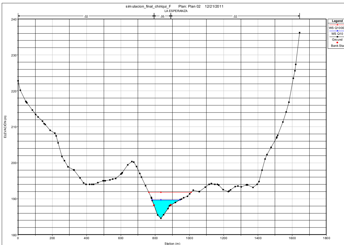
Figura 7: Sección transversal 2K+ 340, vista transversal de la comunidad La Esperanza 26
