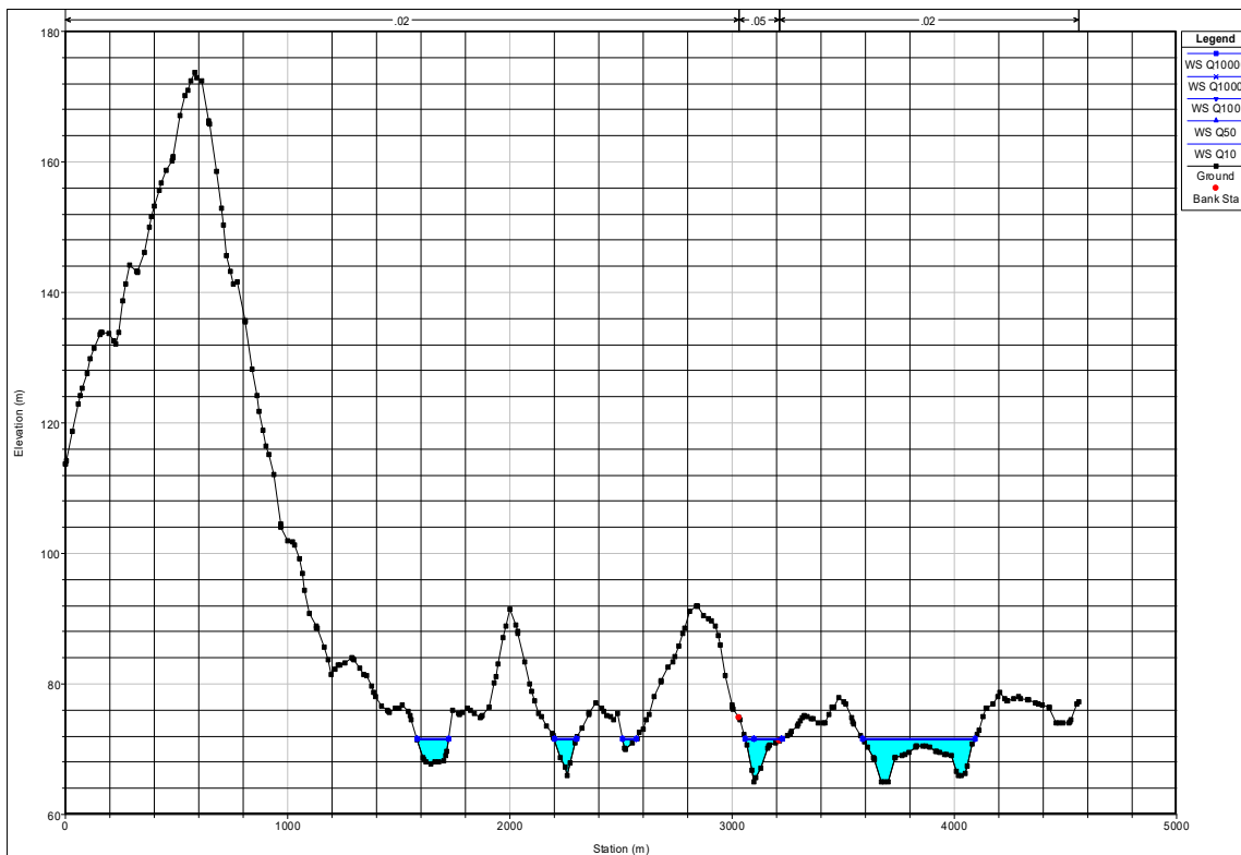
Figura 15: Sección transversal de la comunidad El Higerón para la simulación desde la presa Barrigón 34
