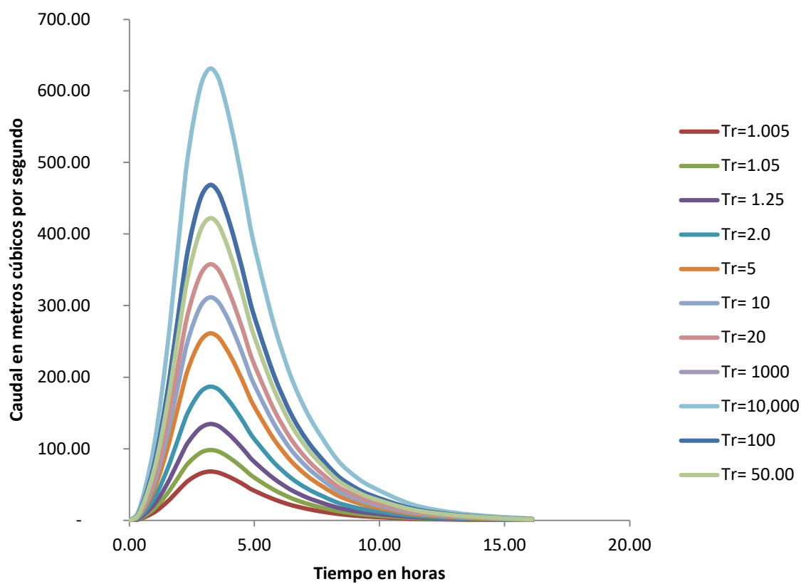
Figura 4. Curvas de caudales con diferentes periodos de retorno para la presa Barrigón 20
