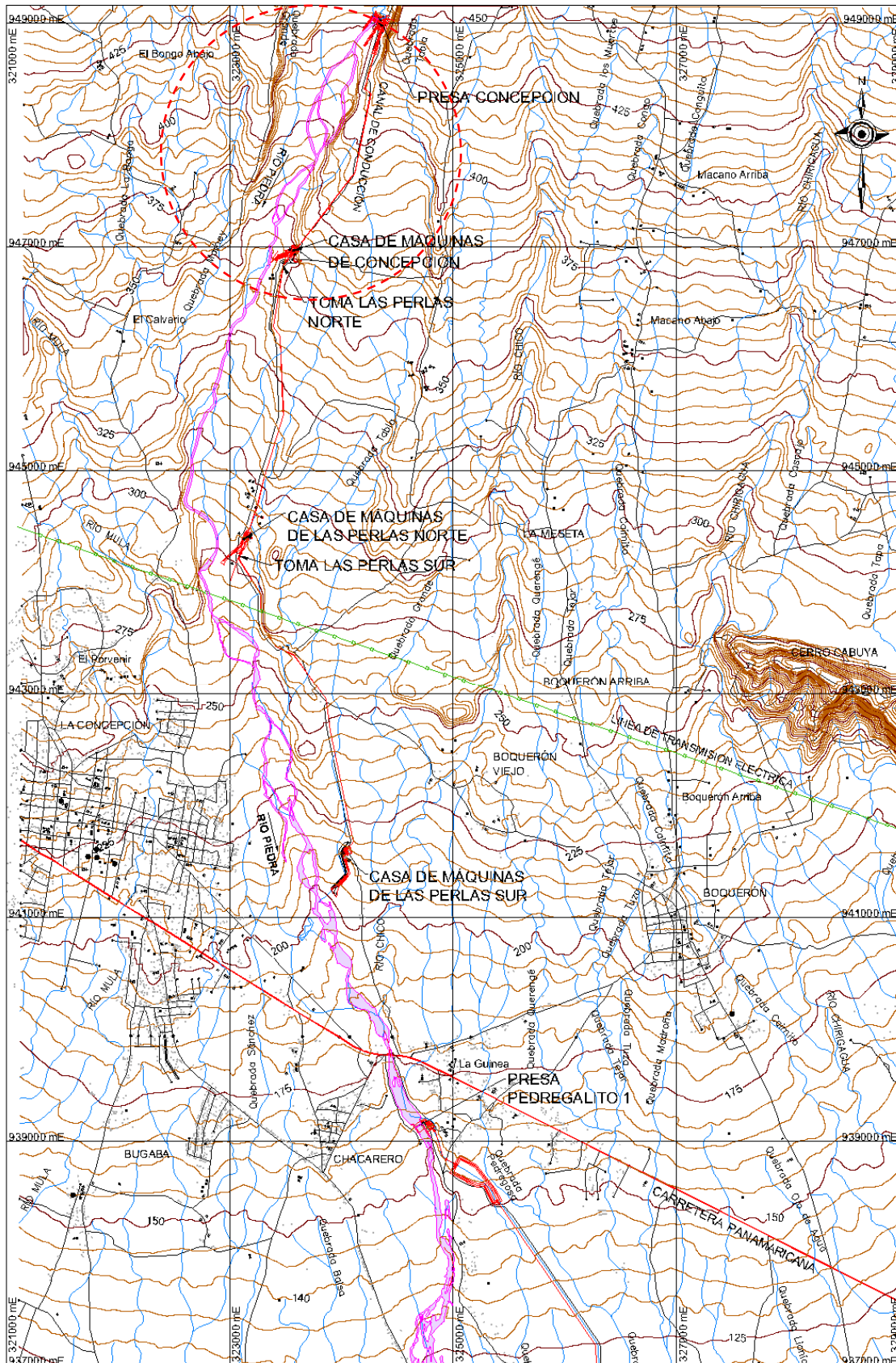
Figura N° 3 – Localización General de la Central Hidroeléctrica Concepción
