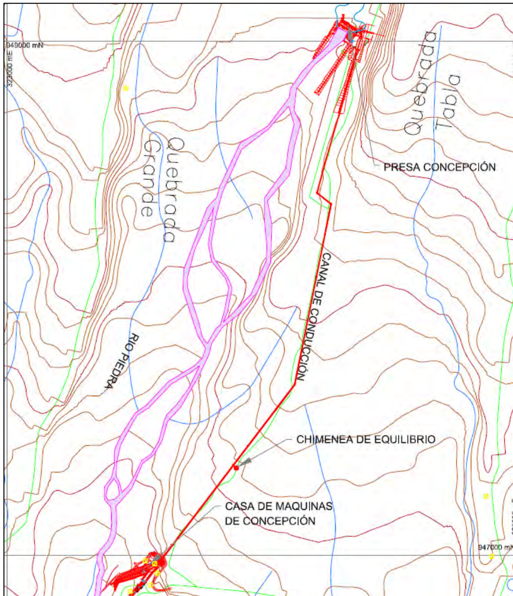
Figura N° 4 - Esquema de la Central Hidroeléctrica Concepción
