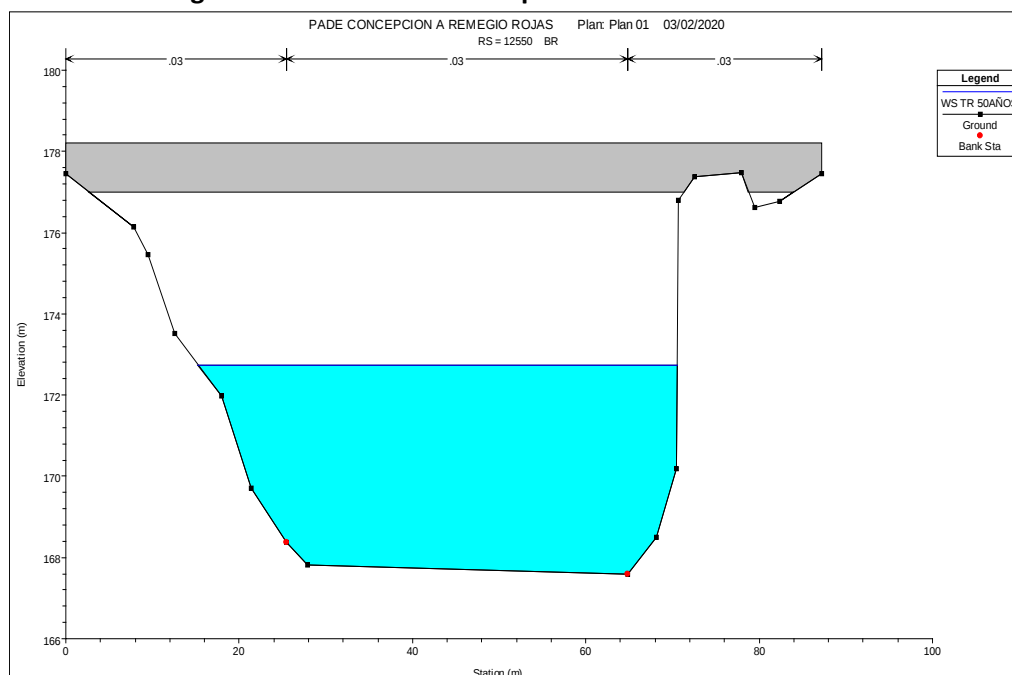
Figura N° D4 - Crecidas en el puente de la Interamericana
