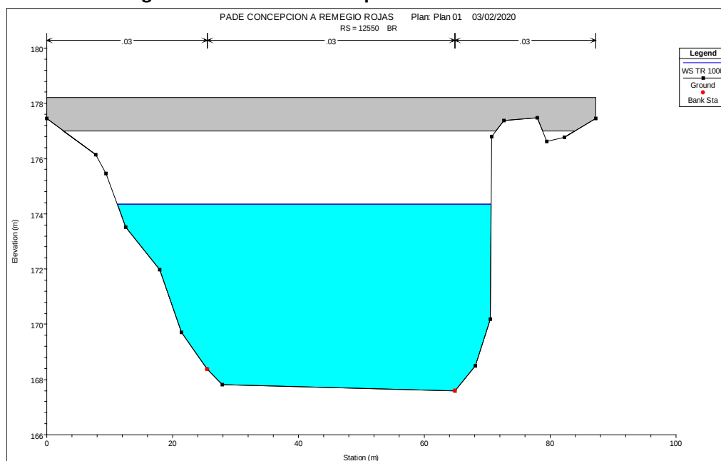
Figura N° 9 - Crecidas en el puente de la Interamericana
