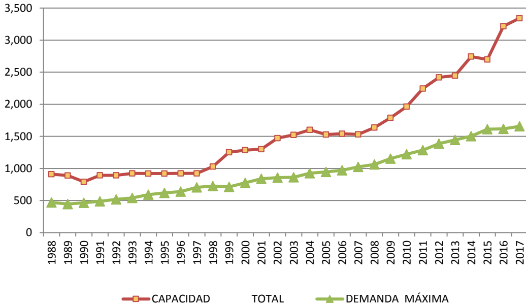
GRÁFICO No. 5 EVOLUCIÓN DE LA CAPACIDAD INSTALADA TOTAL Y DEMANDA MÁXIMA DEL SIN (MW) 1998 - 2017
