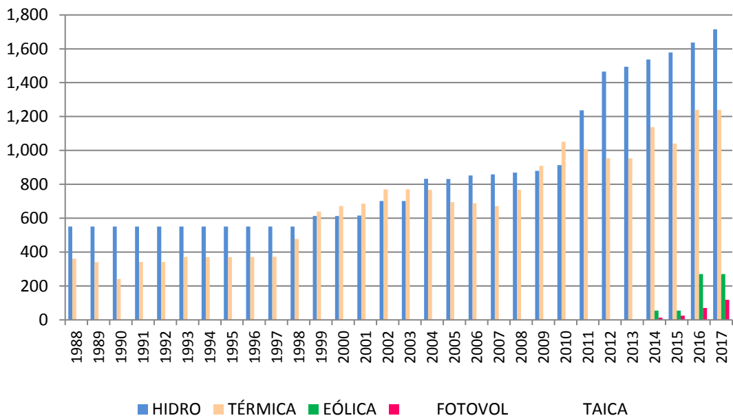
GRÁFICO No. 4 EVOLUCIÓN DE LA CAPACIDAD INSTALADA POR TIPO DE PLANTA (MW) AÑOS 1988 - 2017
