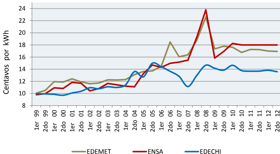
GRÁFICO No. 32 EVOLUCIÓN DEL PRECIO PROMEDIO DE LA ELECTRICIDAD POR SEMESTRE AÑOS 1999 - 2012 (CENTAVOS POR kWh)
