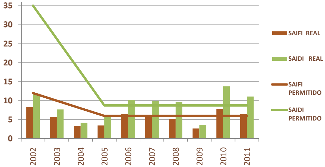
GRÁFICO No. 44 SAIFI Y SAIDI DE EDEMET EN CENTROS URBANOS AÑOS 2002- 2011
