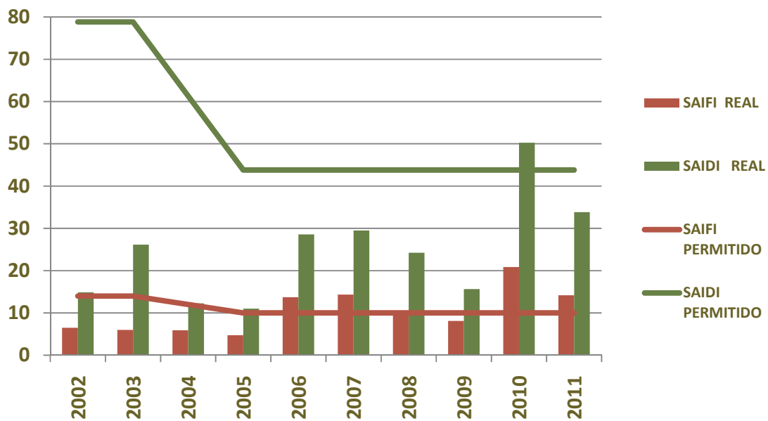
GRÁFICO No. 48 SAIFI Y SAIDI DE EDCHI EN CENTROS RURALES AÑOS 2002 - 2011
