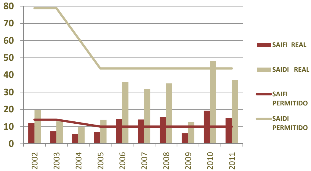
GRÁFICO No. 47 SAIFI Y SAIDI DE EDEMET EN CENTROS RURALES AÑOS 2002 - 2011
