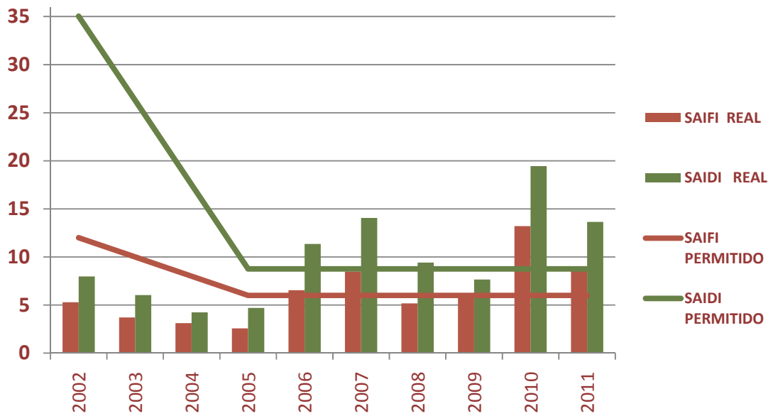
GRÁFICO No. 45 SAIFI Y SAIDI DE EDECHI EN CENTROS URBANOS AÑOS 2002- 2011
