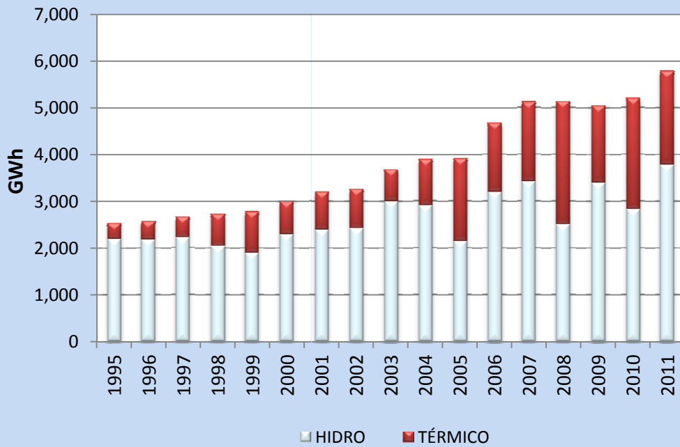
GRÁFICO No. 8 EVOLUCIÓN HISTÓRICA DE LA GENERACIÓN 1995- 2011
