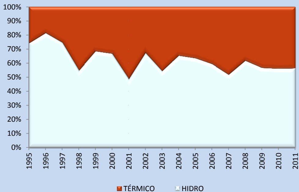
GRÁFICO No. 9 EVOLUCIÓN HISTÓRICA DE LA PARTICIPACIÓN PORCENTUAL DE LA GENERACIÓN POR TIPO DE PLANTA 1995 - 2010
