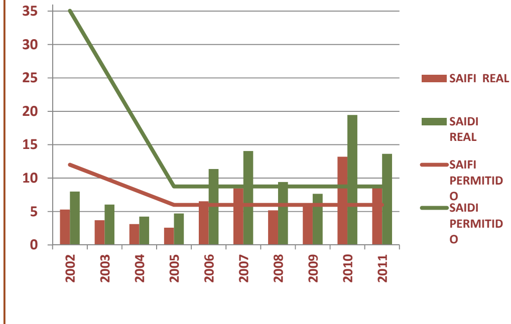
GRÁFICO No. 45 SAIFI Y SAIDI DE EDECHI EN CENTROS URBANOS AÑOS 2002- 2011
