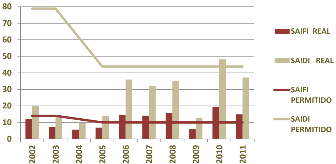
GRÁFICO No. 47 SAIFI Y SAIDI DE EDEMET EN CENTROS RURALES AÑOS 2002 - 2011
