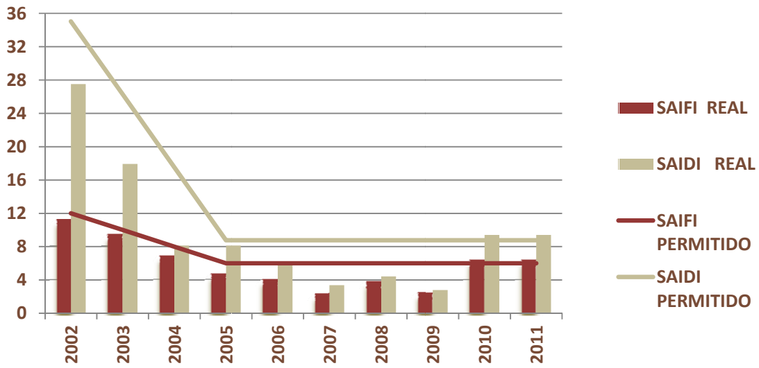
GRÁFICO No. 43 SAIFI Y SAIDI DE ELEKTRA EN CENTROS URBANOS AÑOS 2002- 2011
