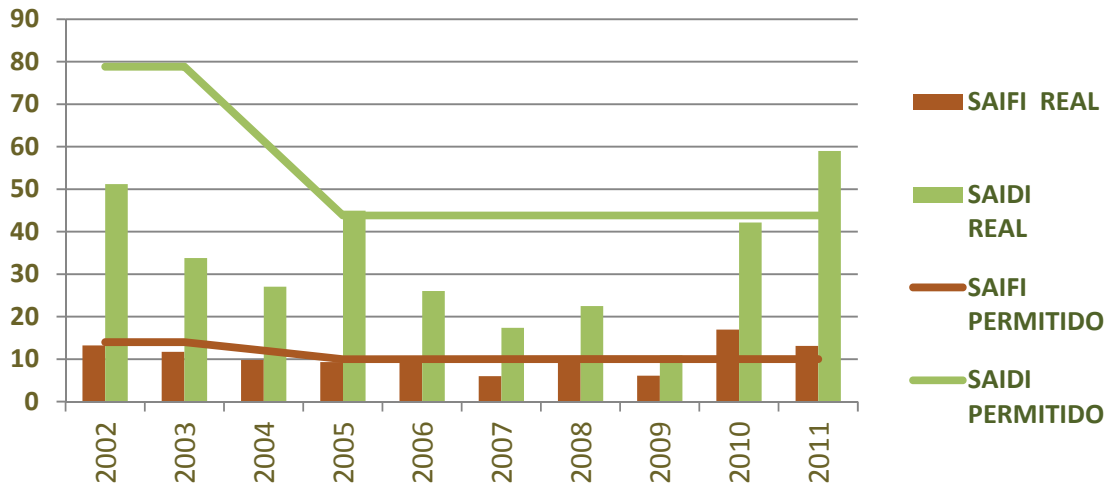
GRÁFICO No. 46 SAIFI Y SAIDI DE ELEKTRA EN CENTROS RURALES AÑOS 2002 - 2011
