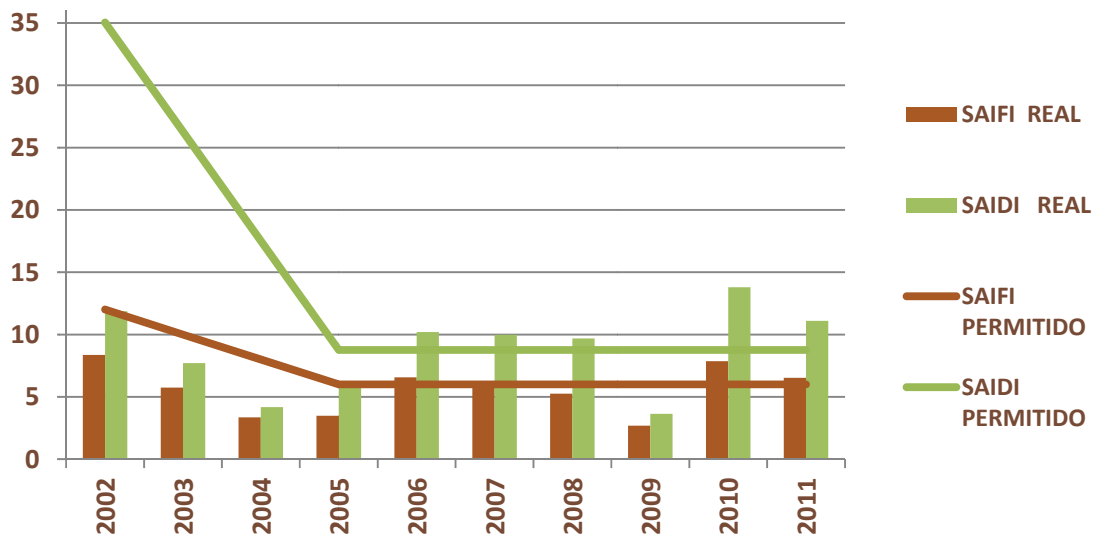
GRÁFICO No. 44 SAIFI Y SAIDI DE EDEMET EN CENTROS URBANOS AÑOS 2002- 2011
