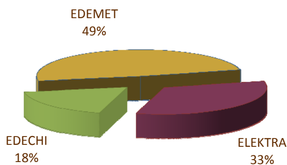
GRÁFICO No. 13 PORCENTAJE DE LA LONGITUD DE LÍNEAS DE DISTRIBUCIÓN POR EMPRESA 2009
