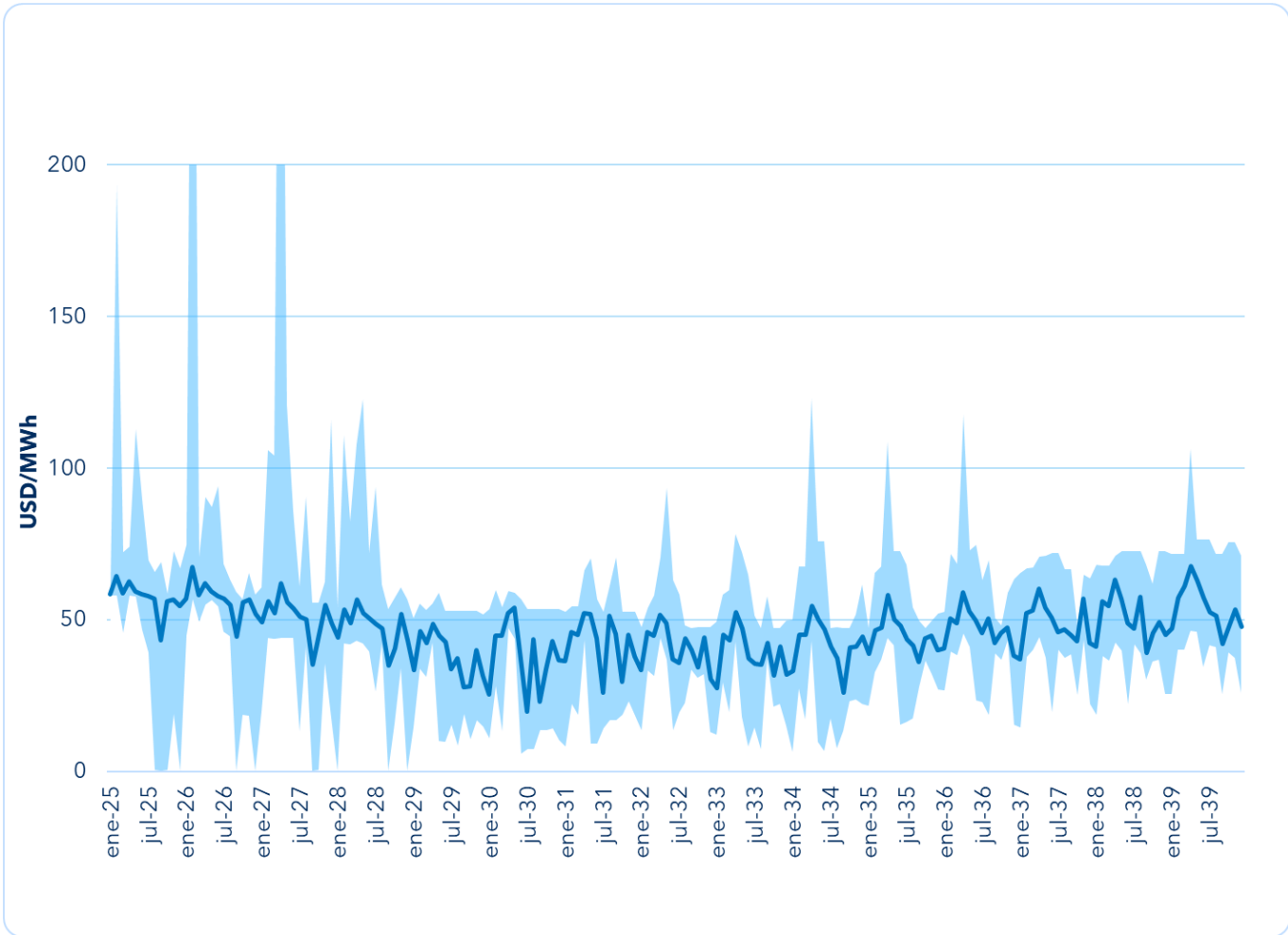
Gráfico A1. 2 Costos Marginales del Escenario Referencia A1
