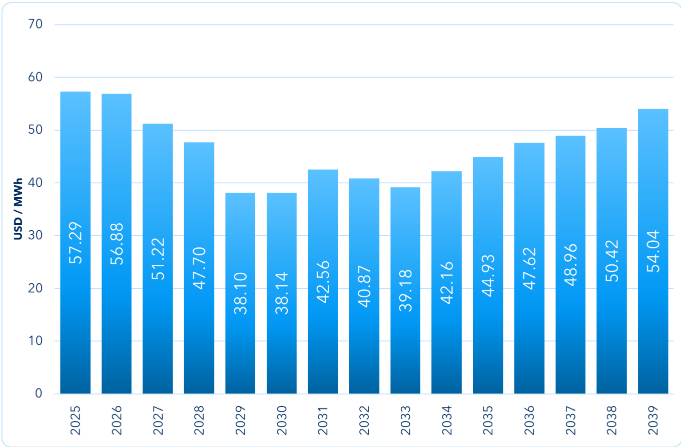
Gráfico A1. 3 Costos Marginales del Escenario Referencia A1
