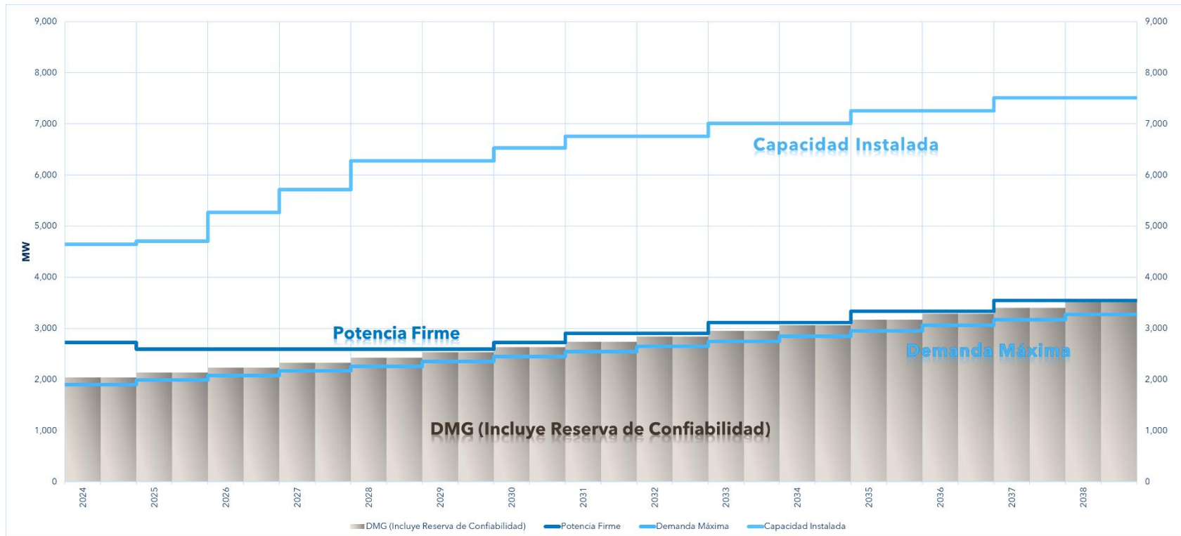
Gráfico A1. 1 Balance de Potencia vs Demanda del Escenario Referencia A1
