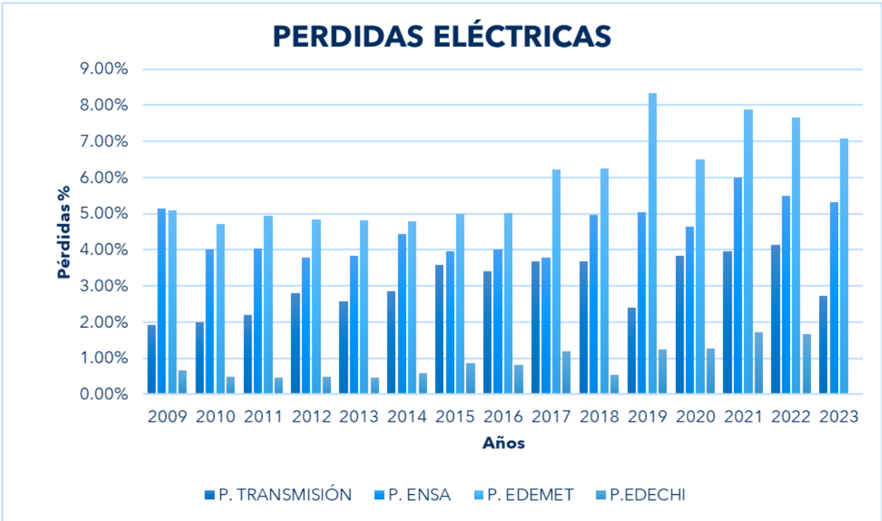
CUADRO NO.10: PÉRDIDAS POR DISTRIBUIDORA Y TOTAL.
