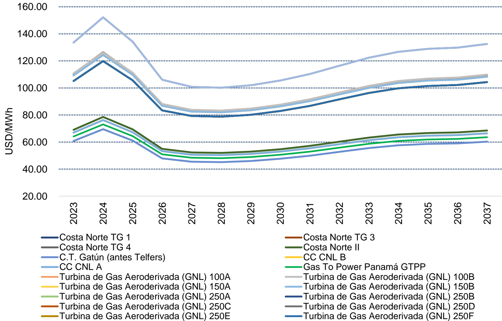
Gráfico N° A4.5: Costo Variable de Producción Plantas de Gas Natural Plan Indicativo de Generación 2023-2037.
