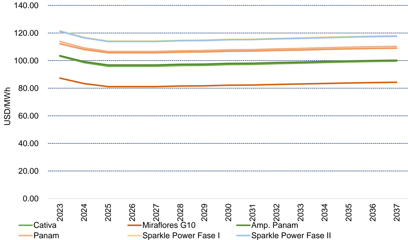
Gráfico N° A4.3: Costo Variable de Producción Plantas de Bunker C Plan Indicativo de Generación 2023-2037.
