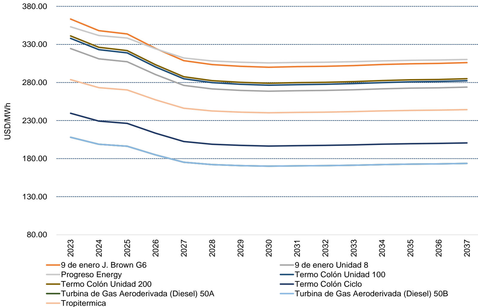
Gráfico N° A4.2: Costo Variable de Producción Plantas de Diésel Plan Indicativo de Generación 2023-2037.
