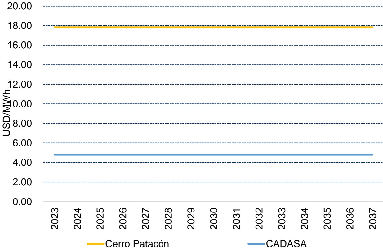
Gráfico N° A4.4: Costo Variable de Producción Plantas de Bagazo y Metano Plan Indicativo de Generación 2023-2037.
