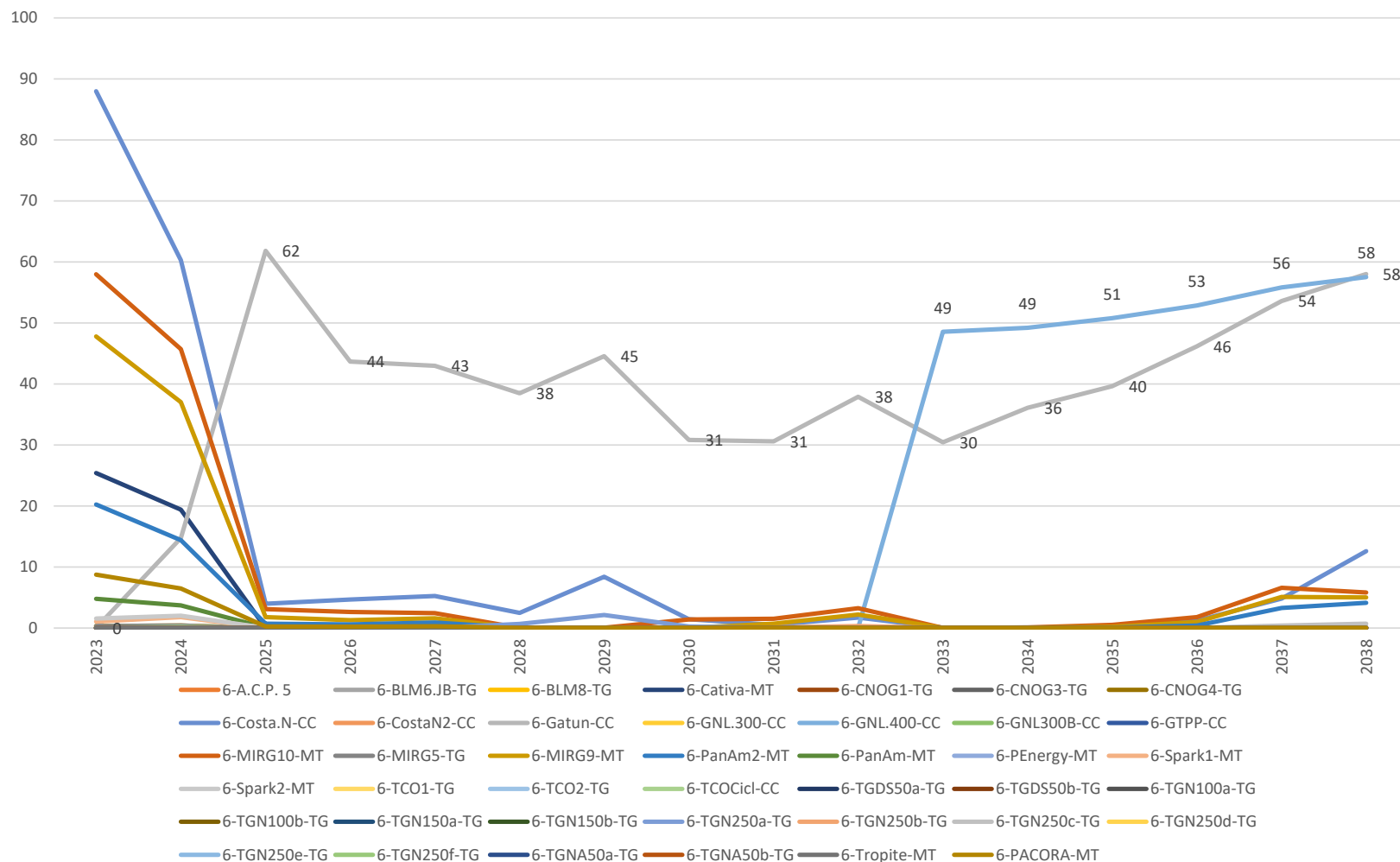
Gráfico N° A4.6: Factor de Planta de las Plantas Térmicas del Escenario de Tendencial.
