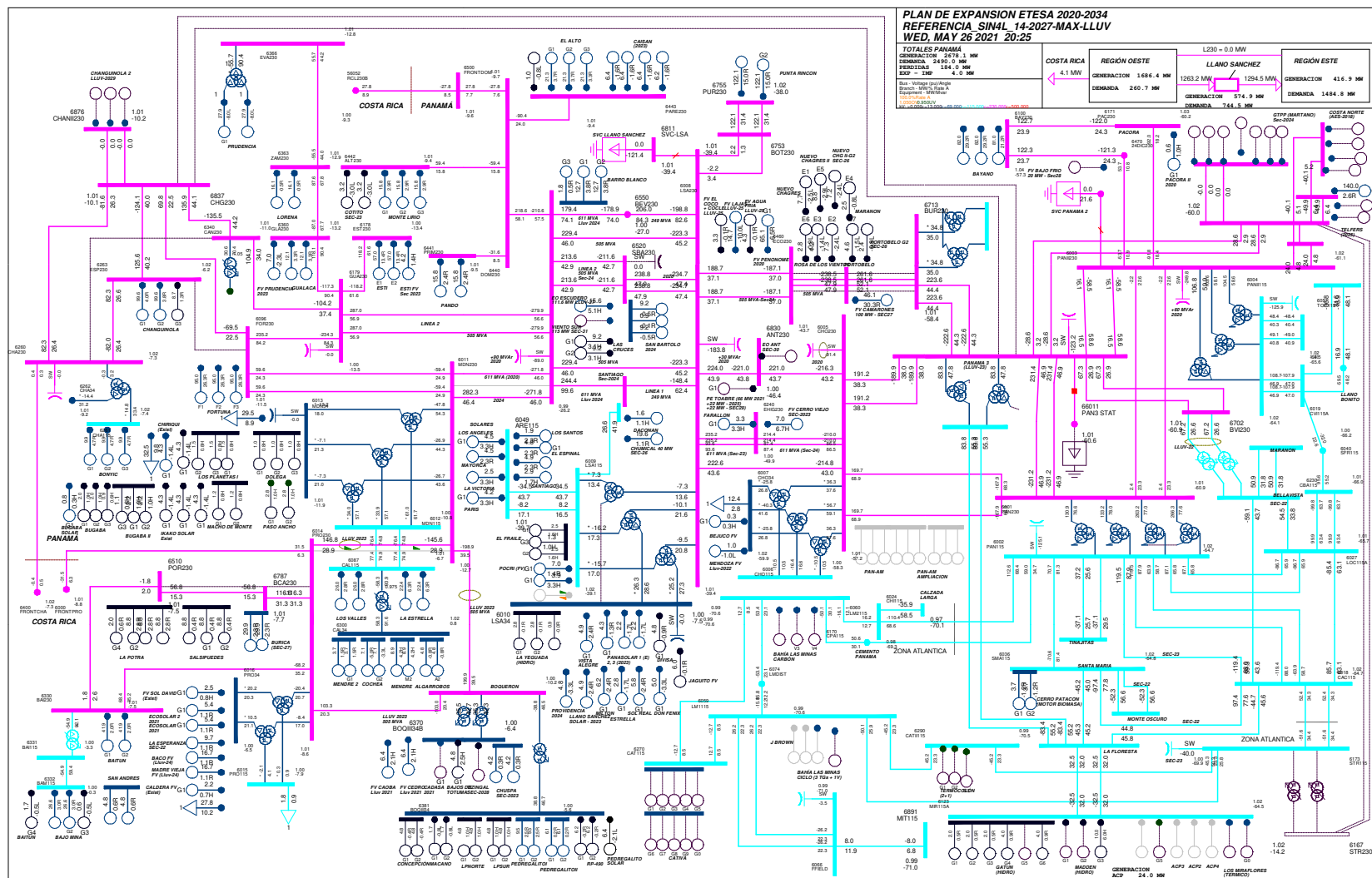
Gráfico 17. Escenario Referencia_Sin4L_14-2027-Max-Lluv. Flujo con red completa
