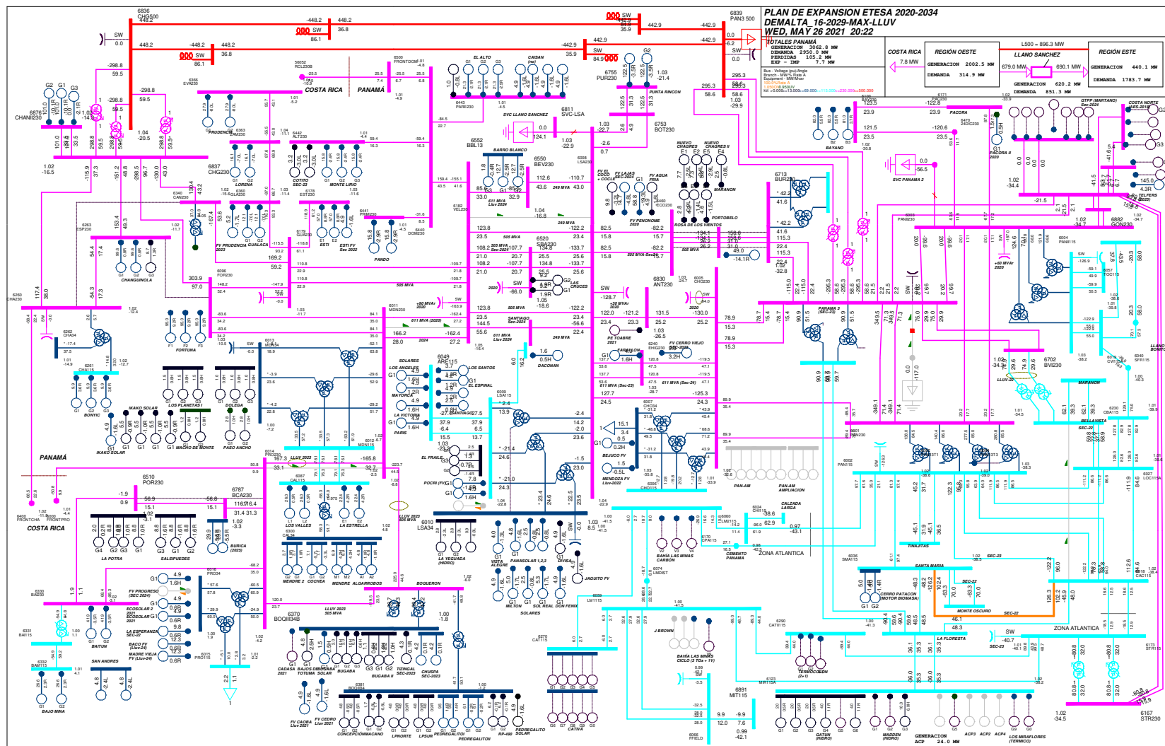
Gráfico 6. Escenario DemAlta_16-2029-Max-Lluv. Flujo con red completa
