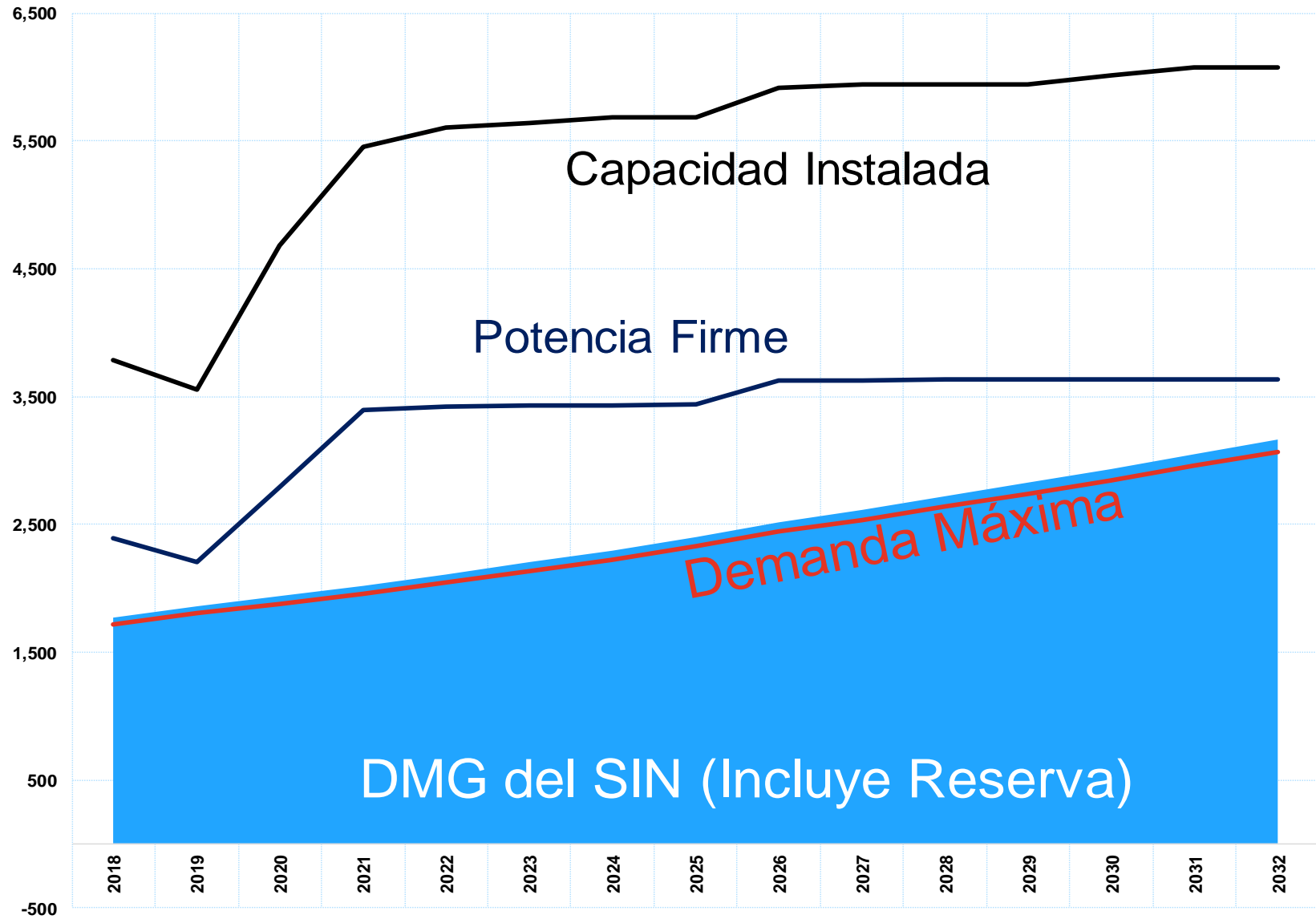
Gráfico N° A2.1 Balance de Potencia vs Demanda del Alternativo I
