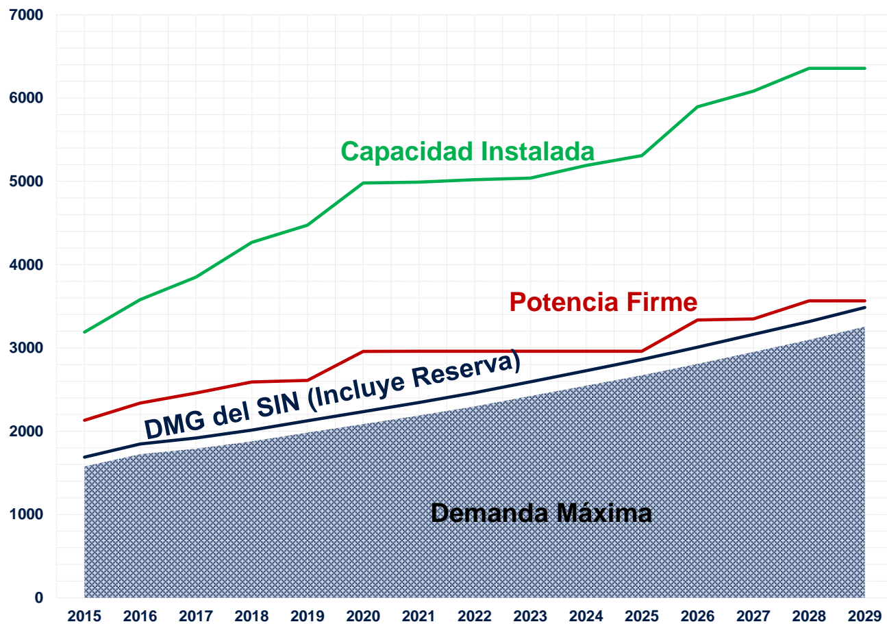
Gráfico N° A3.1 Balance de Potencia vs Demanda del Escenario de Renovables
