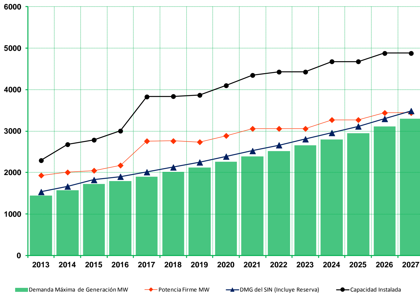
Gráfico N° A3.1 Balance de Potencia vs Demanda del Caso REGMHTTLA13
