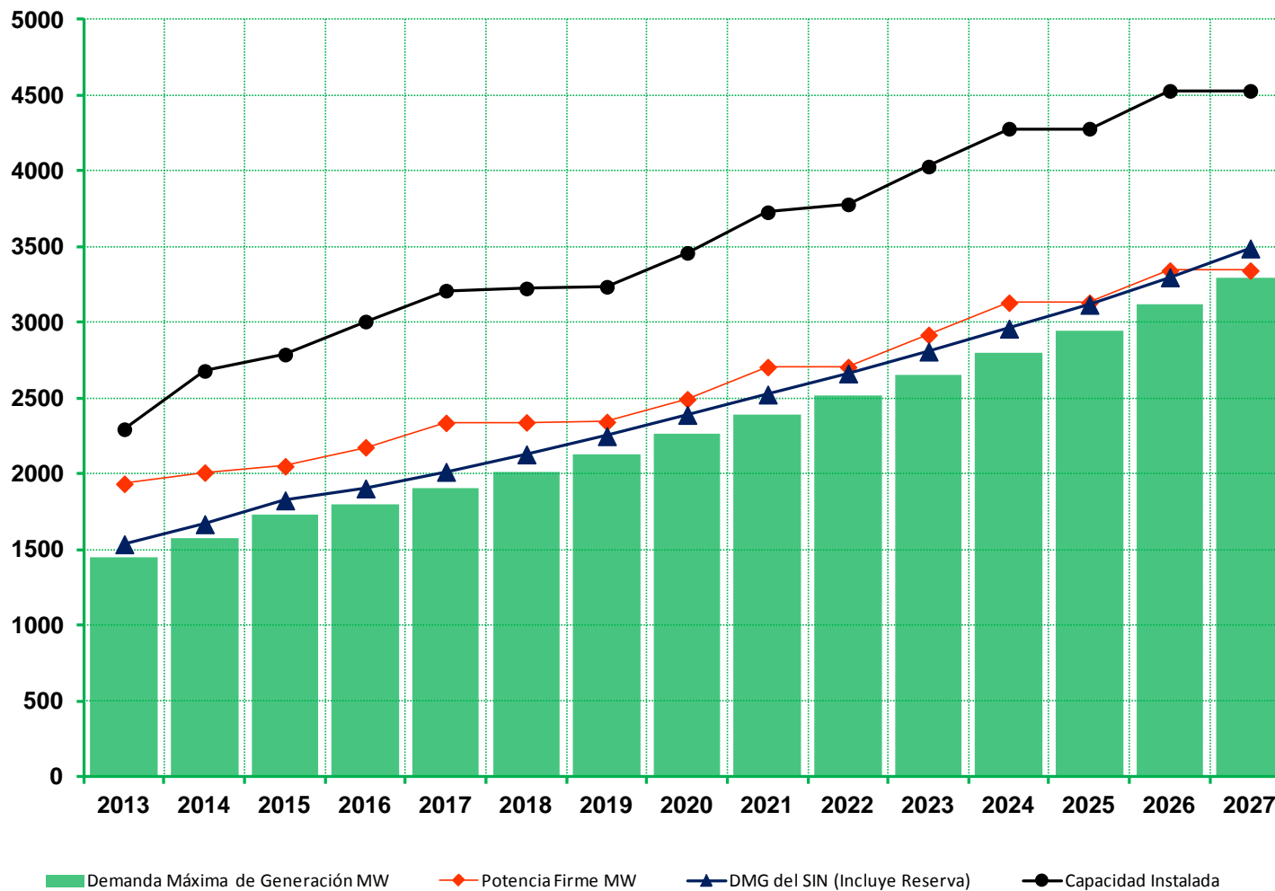
Gráfico N° A2.1 Balance de Potencia vs Demanda del Caso REGMHTCB13
