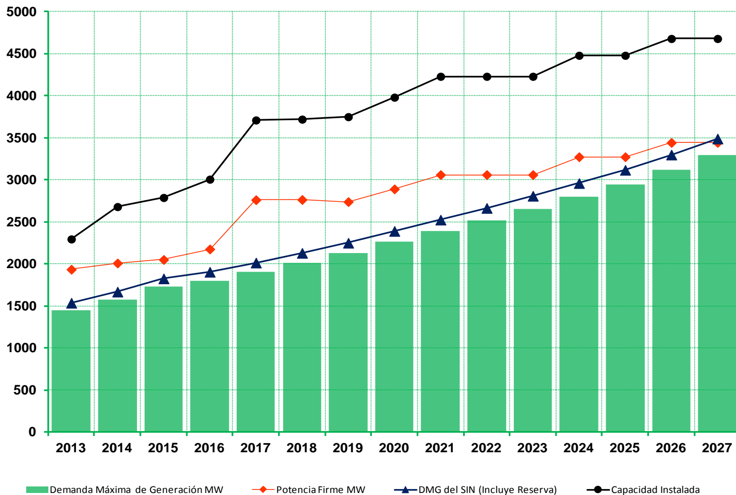
Gráfico N° A1.1 Balance de Potencia vs Demanda del Caso REGMHTGNC13
