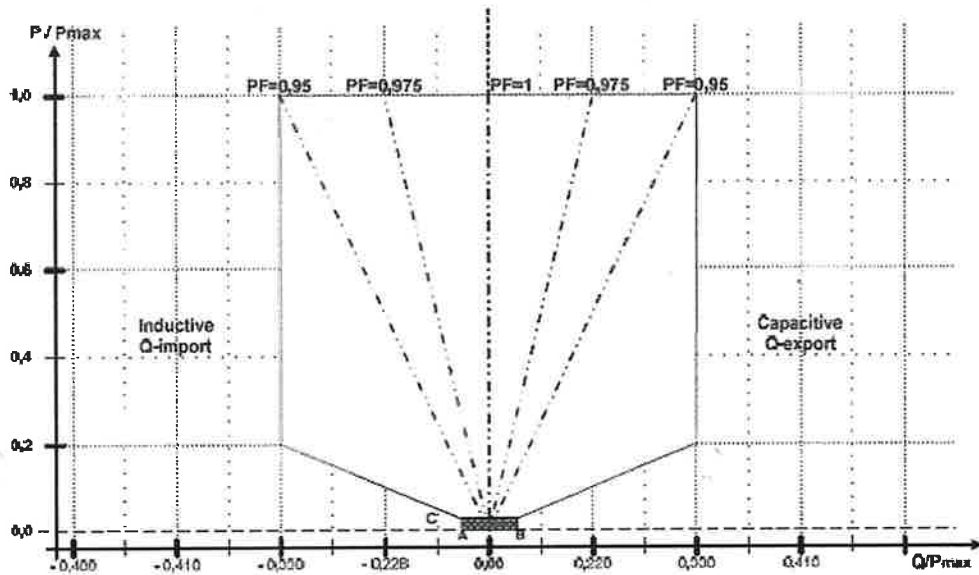
Figura B.3.1. Requisitos para la Potencia Reactiva.
