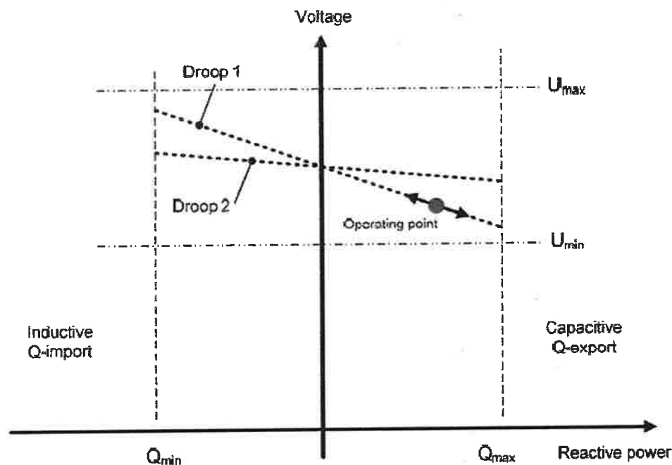
Figura B.4.3. Control de Voltaje.
