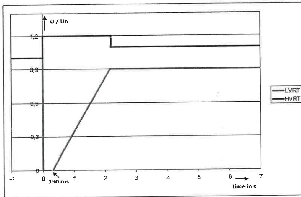
Figura B.1.2. Requerimientos de Alto Voltaje (LVRT) y Bajo Voltaje (HVRT).
