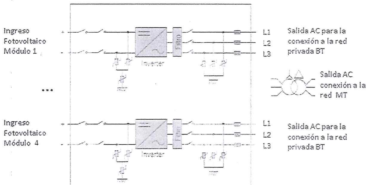
Figura 1 - Esquema de bloques del inversor
