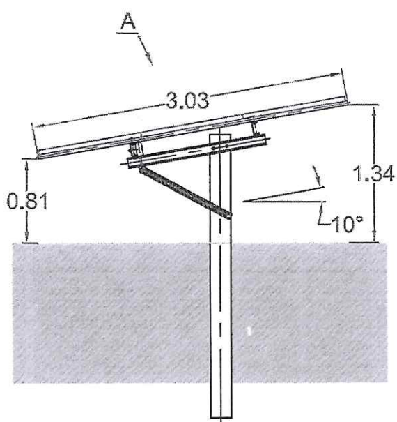
Figura 3 – Estructura, vista lateralmente
