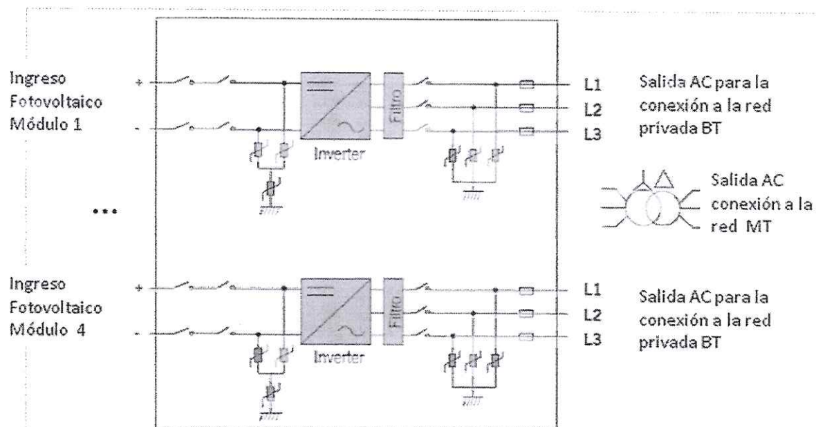
Figura 1 - Esquema de bloques del inversor
