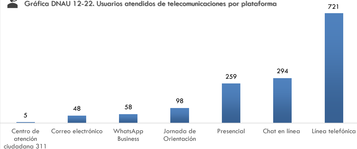
Gráfica DNAU 12-22. Usuarios atendidos de telecomunicaciones por plataforma
